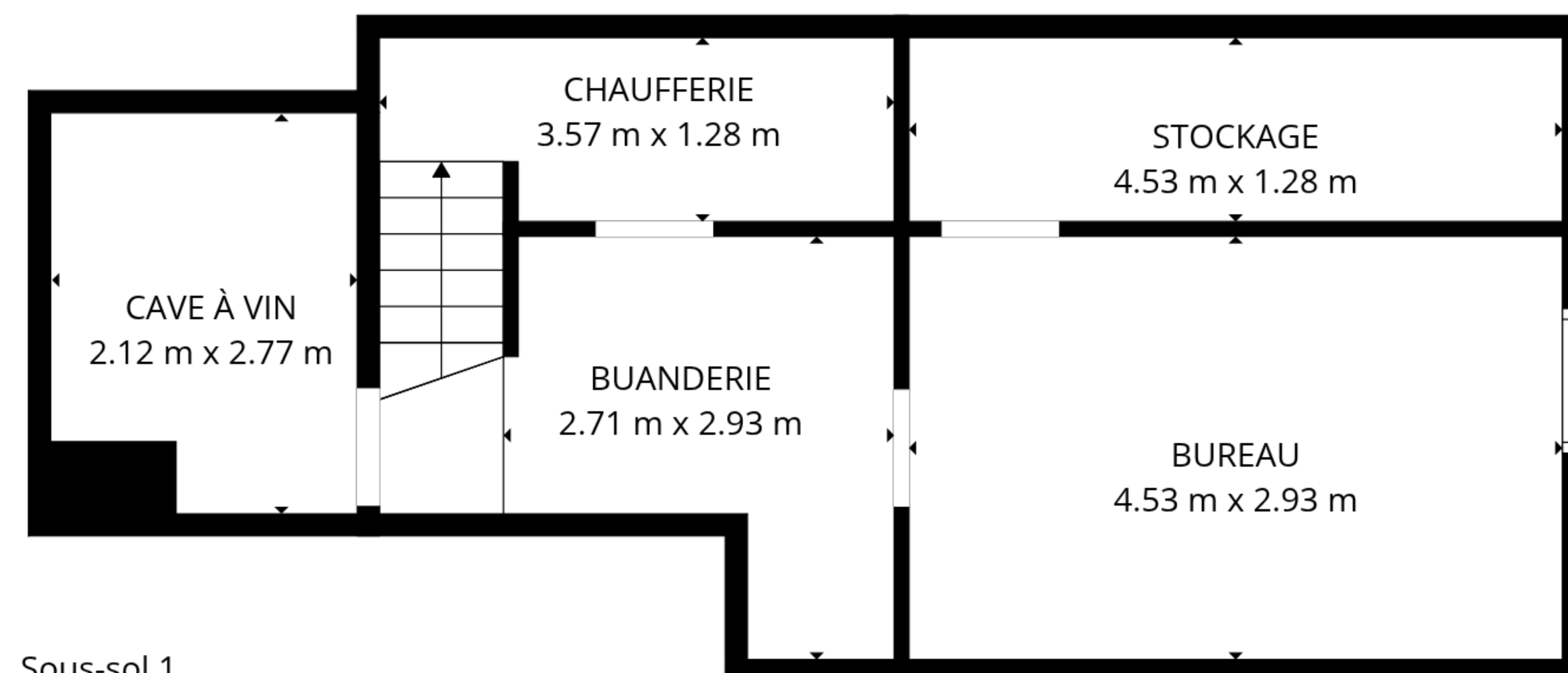
Sous-sol 1
