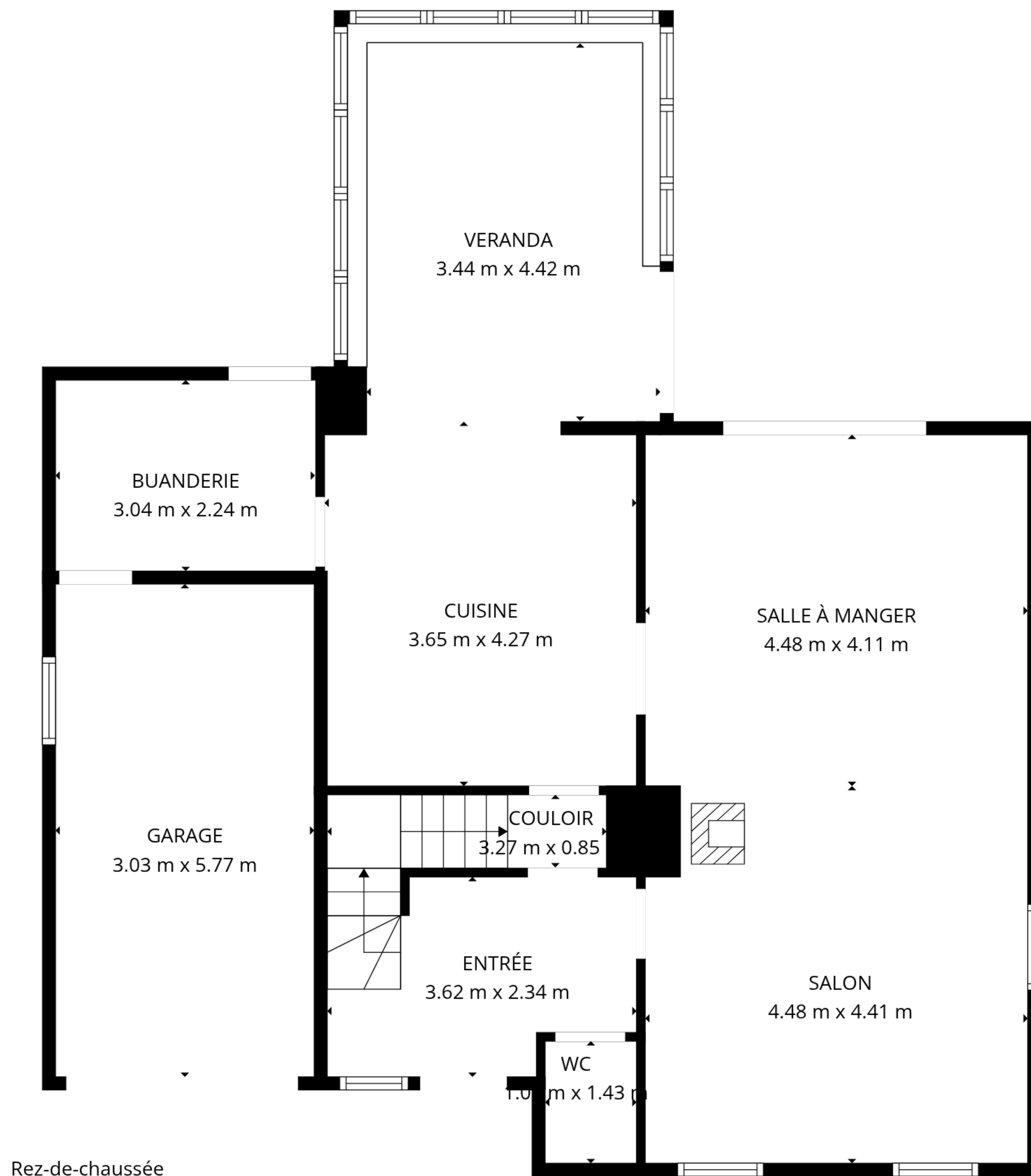
Rez-de-chaussée
