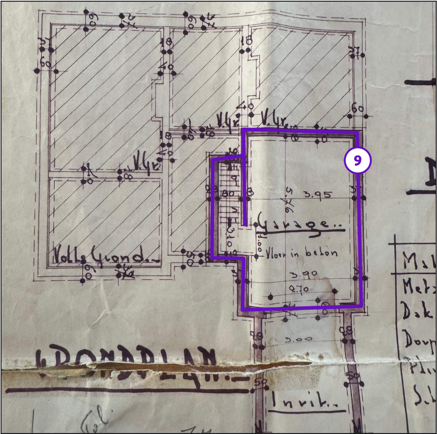
Legende van plan 1.7: -1 verdieping
