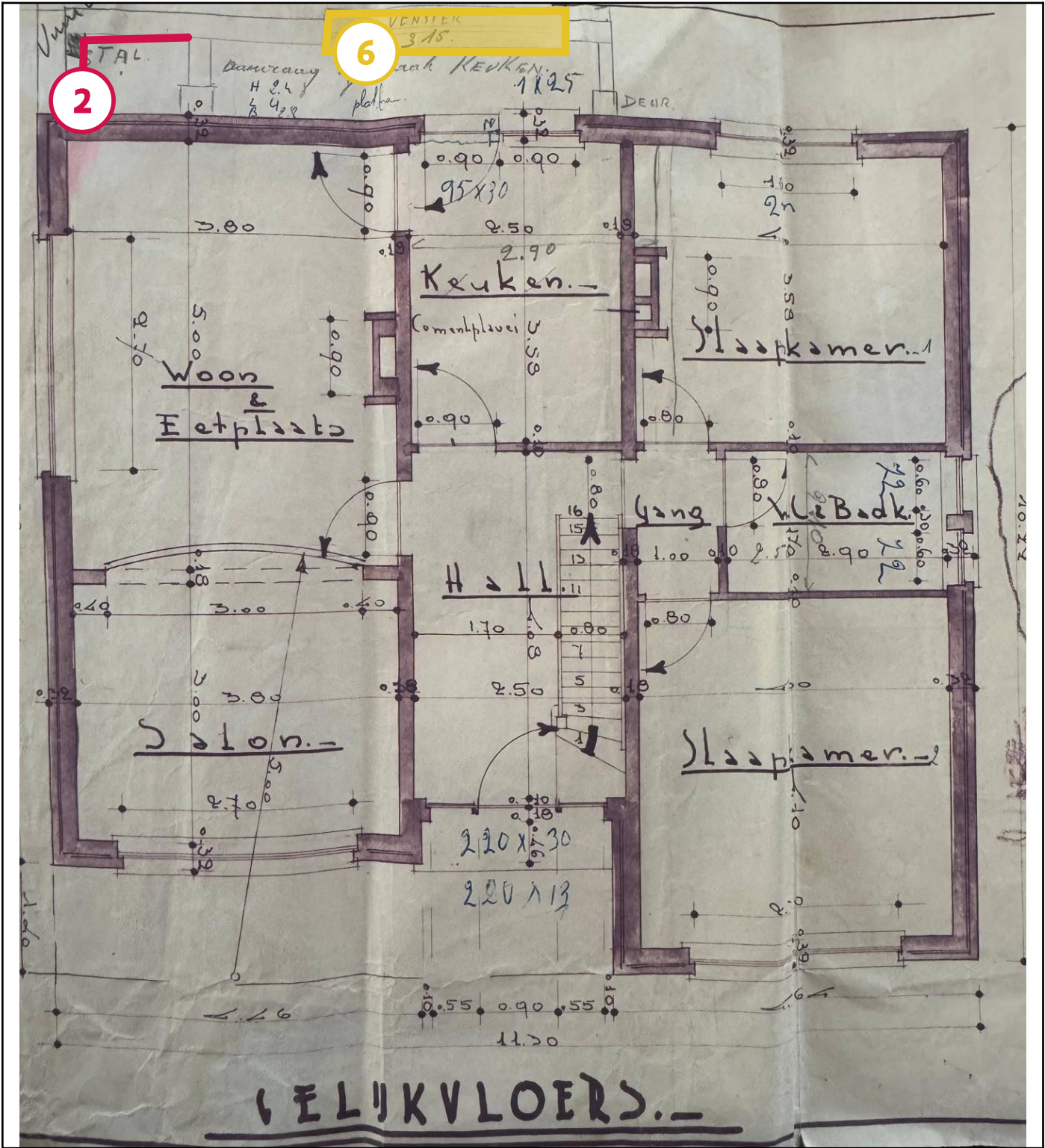
Legende van plan 1.11: Gelijkvloers
