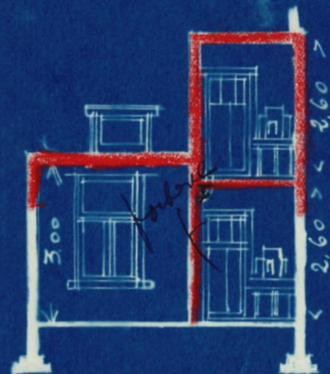
doorsnede AB
