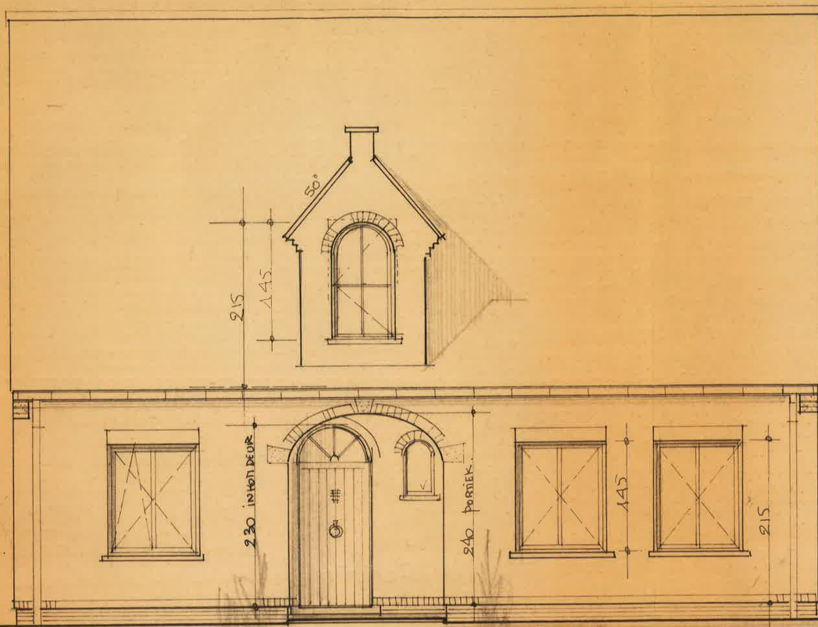
VOORGEVEL
