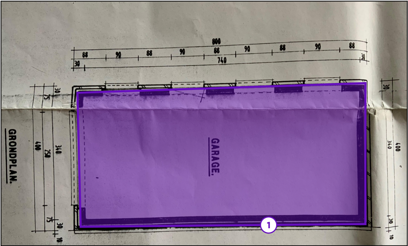
Legende van plan 2.1: Grondplan glv
