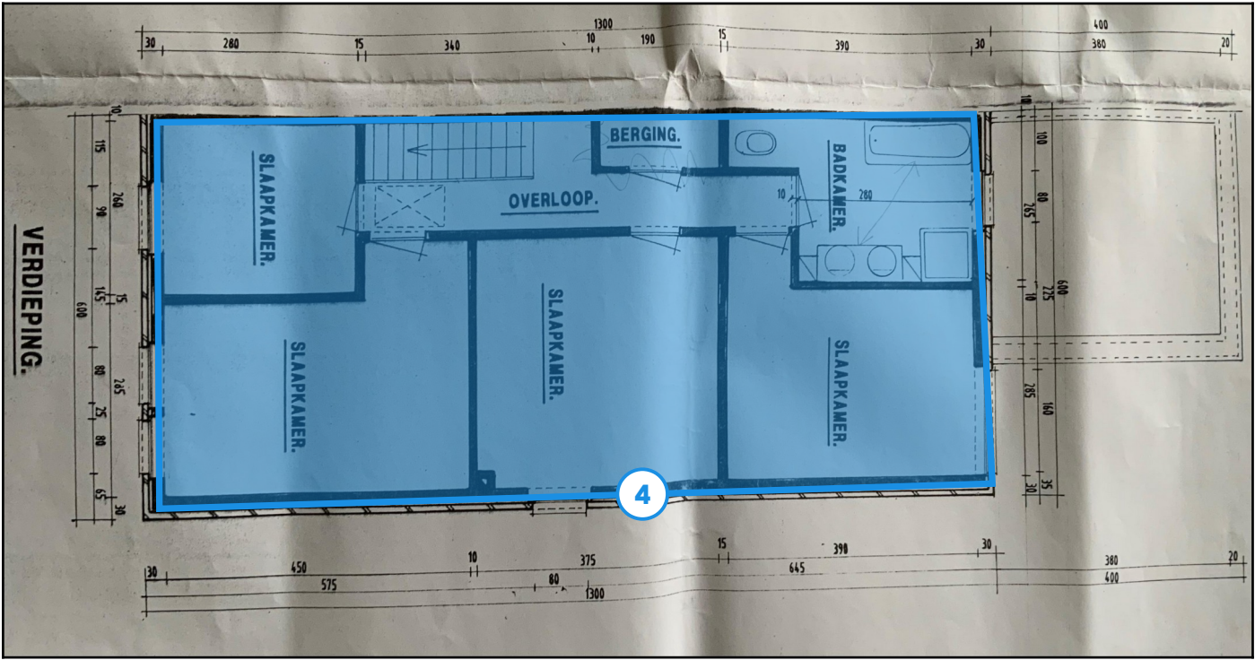
Legende van plan 1.4: Grondplan 1v
