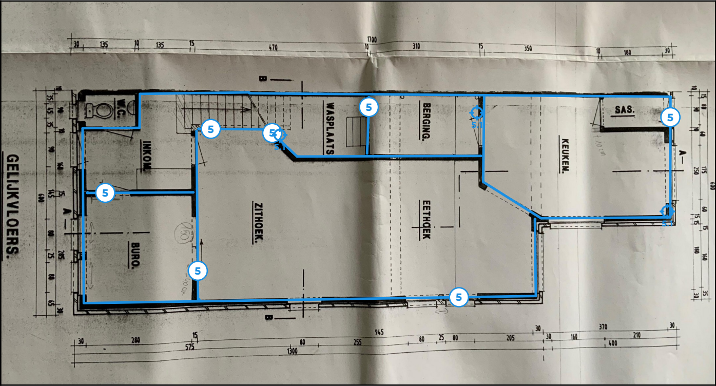
Legende van plan 1.1: Grondplan glv
