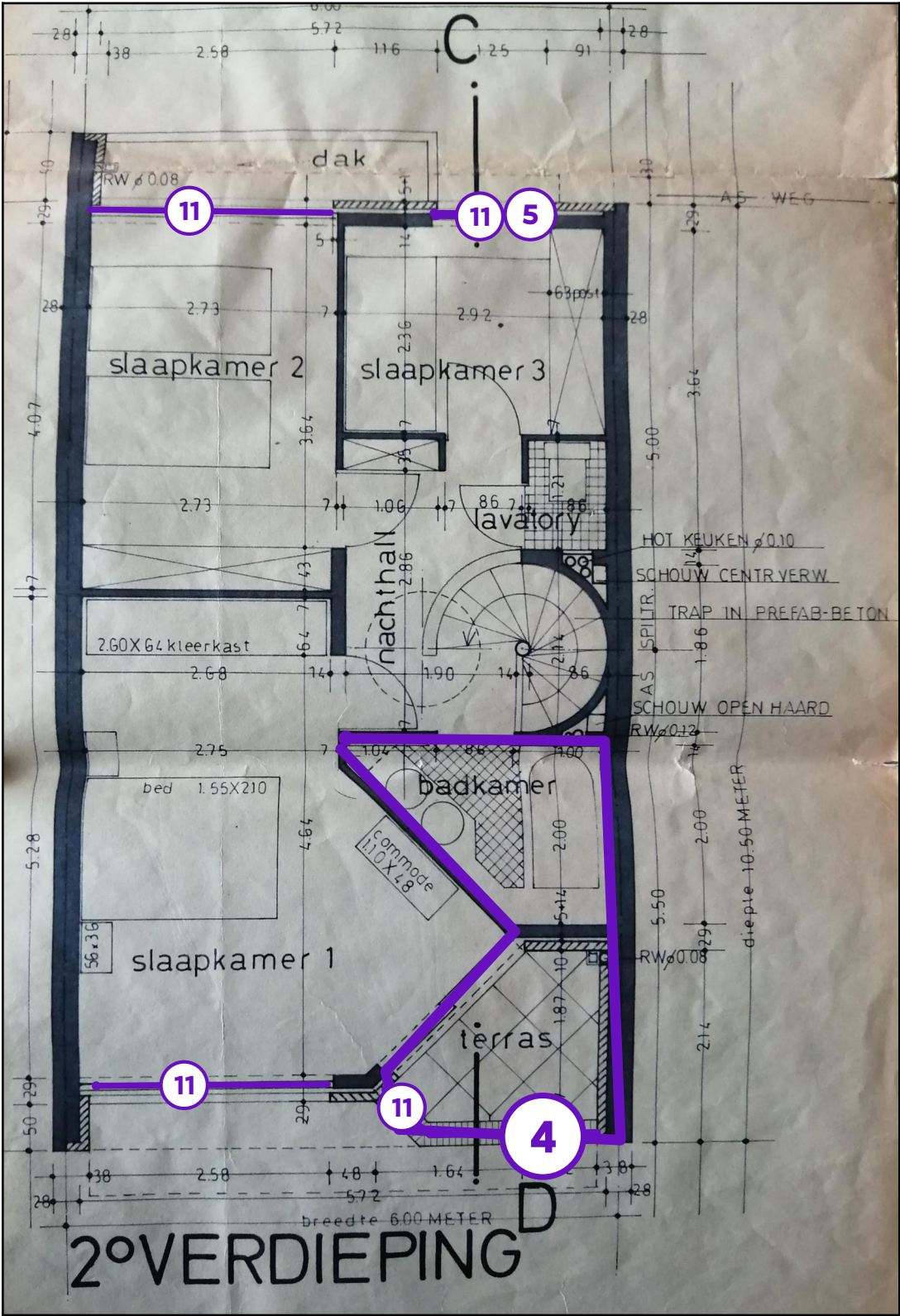
Legende van plan 1.4: grondplan verdieping 2
