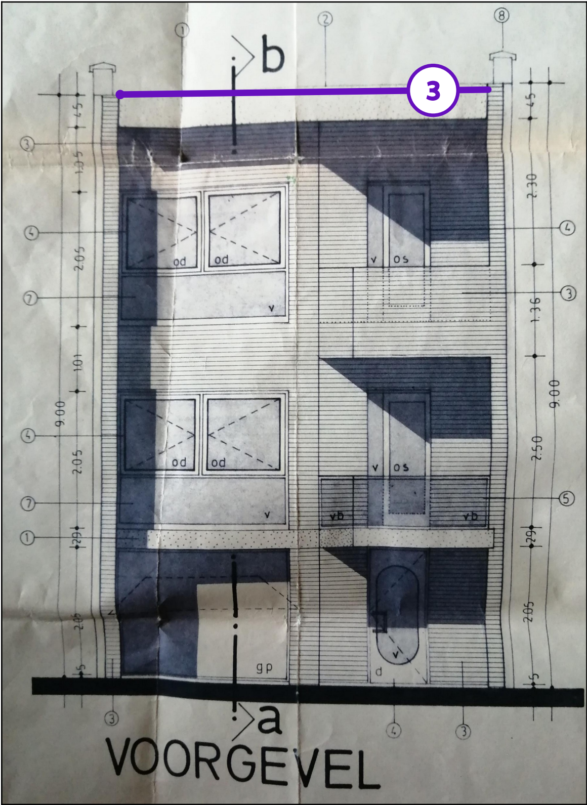
Legende van plan 1.8: gevel voor
