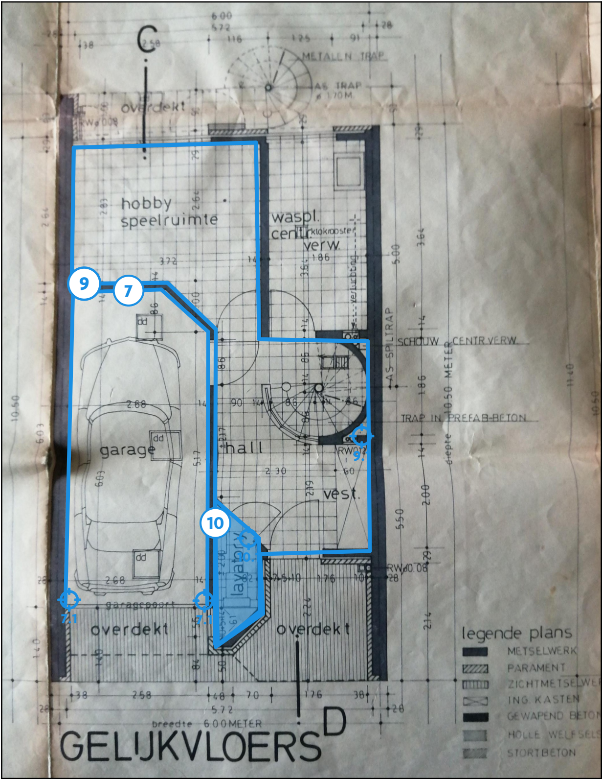
Legende van plan 1.5: gipsplan gelijkvloers
