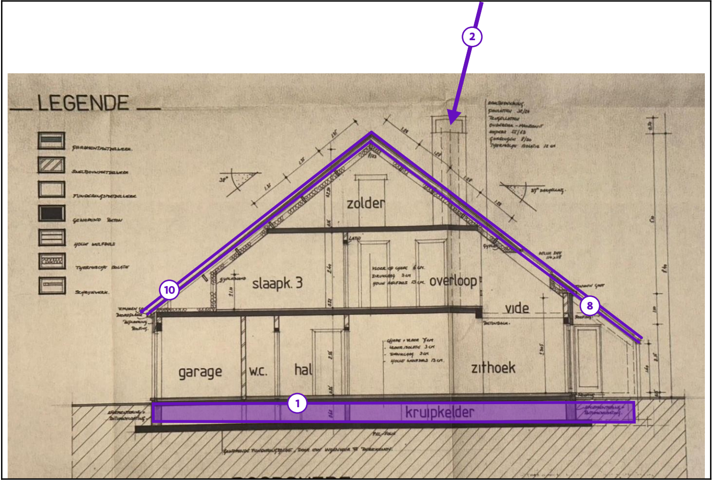
Legende van plan 1.5: zij aanzicht
