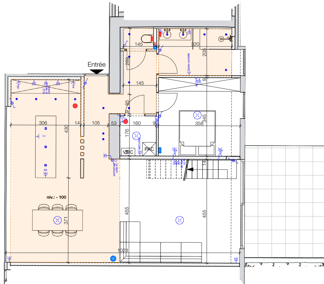
Rez-de-chaussée 1:100
