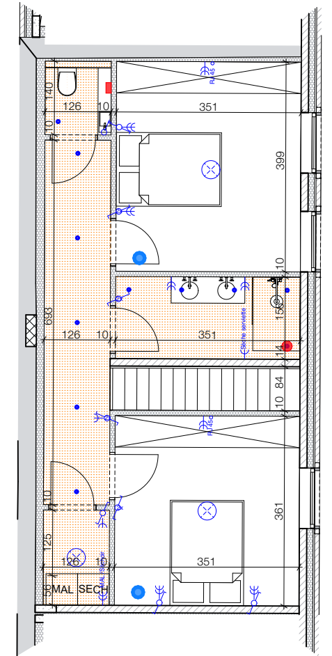
1er étage 1:100
