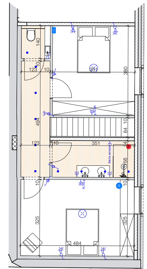
1er étage 1:100
