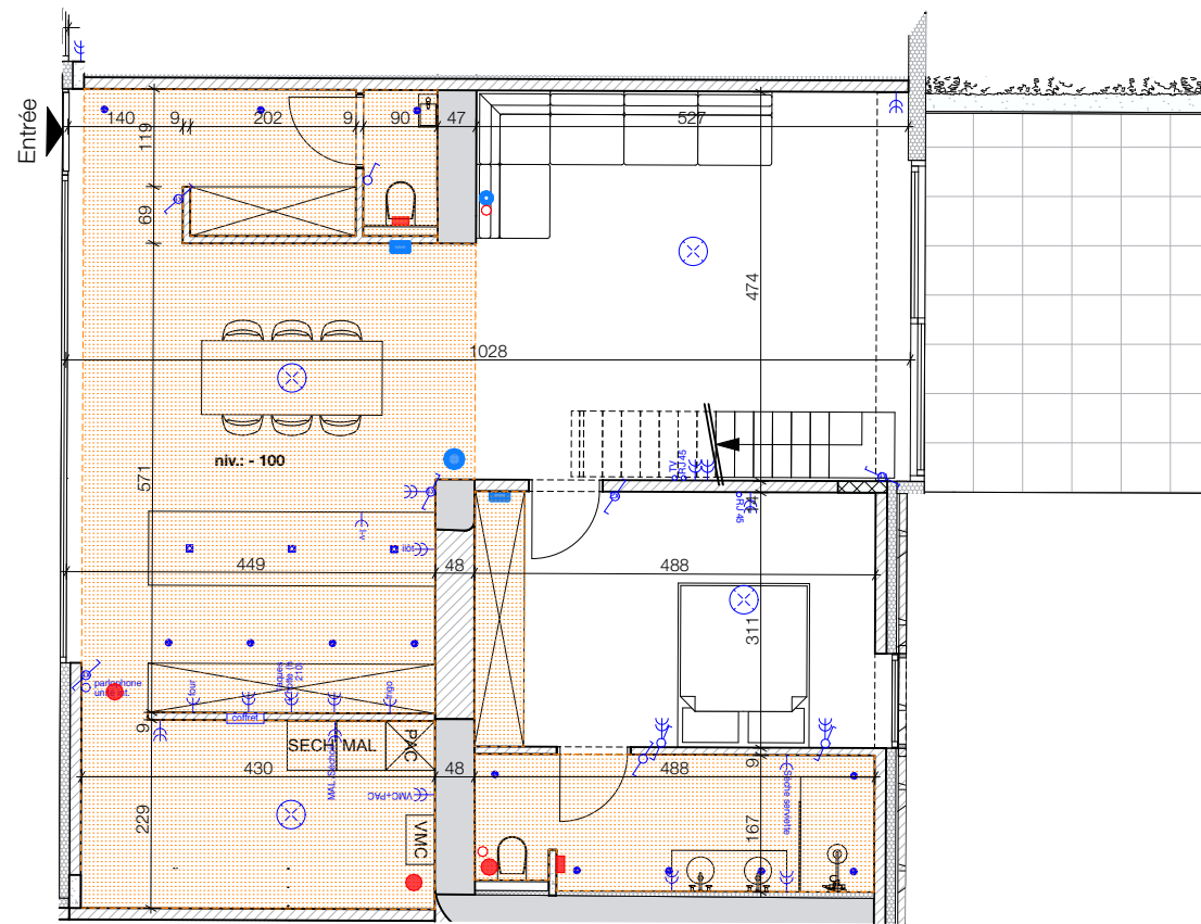
Rez-de-chaussée 1:100
