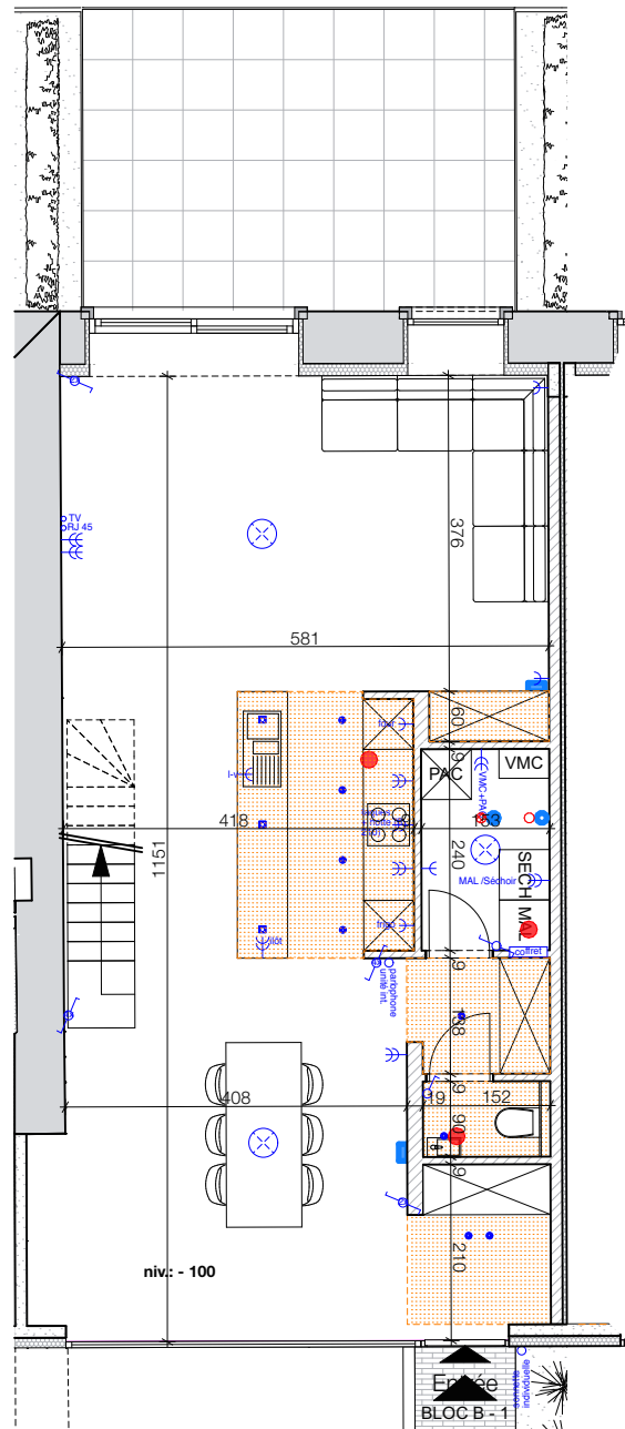
Rez-de chaussée 1:100
