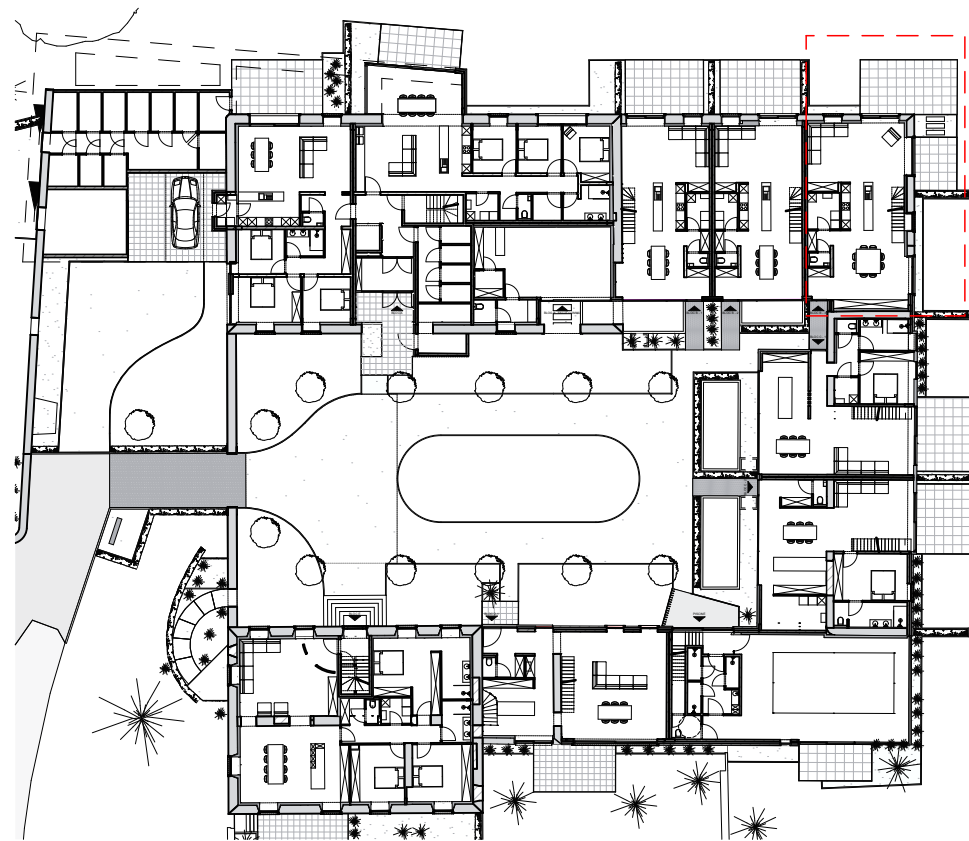
Rez-de-chaussée
