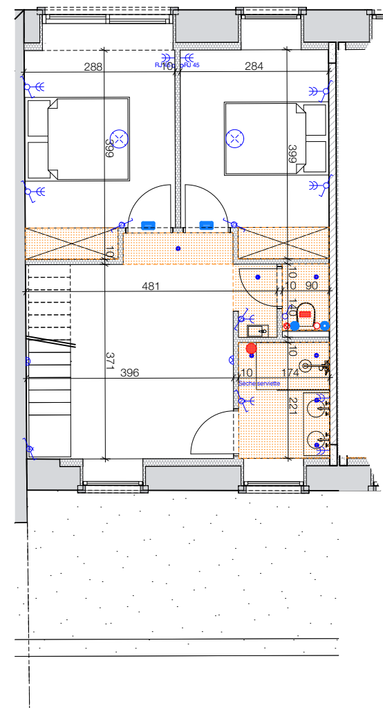
1er étage 1:100
