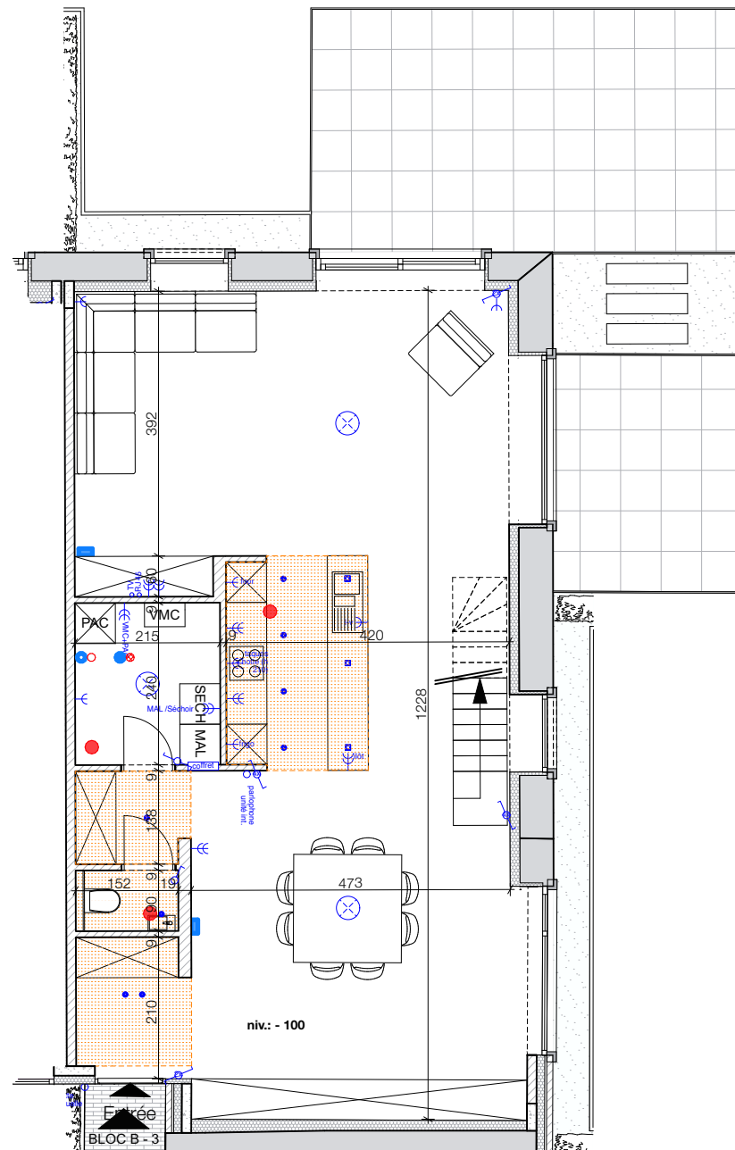
Rez-de-chaussée
