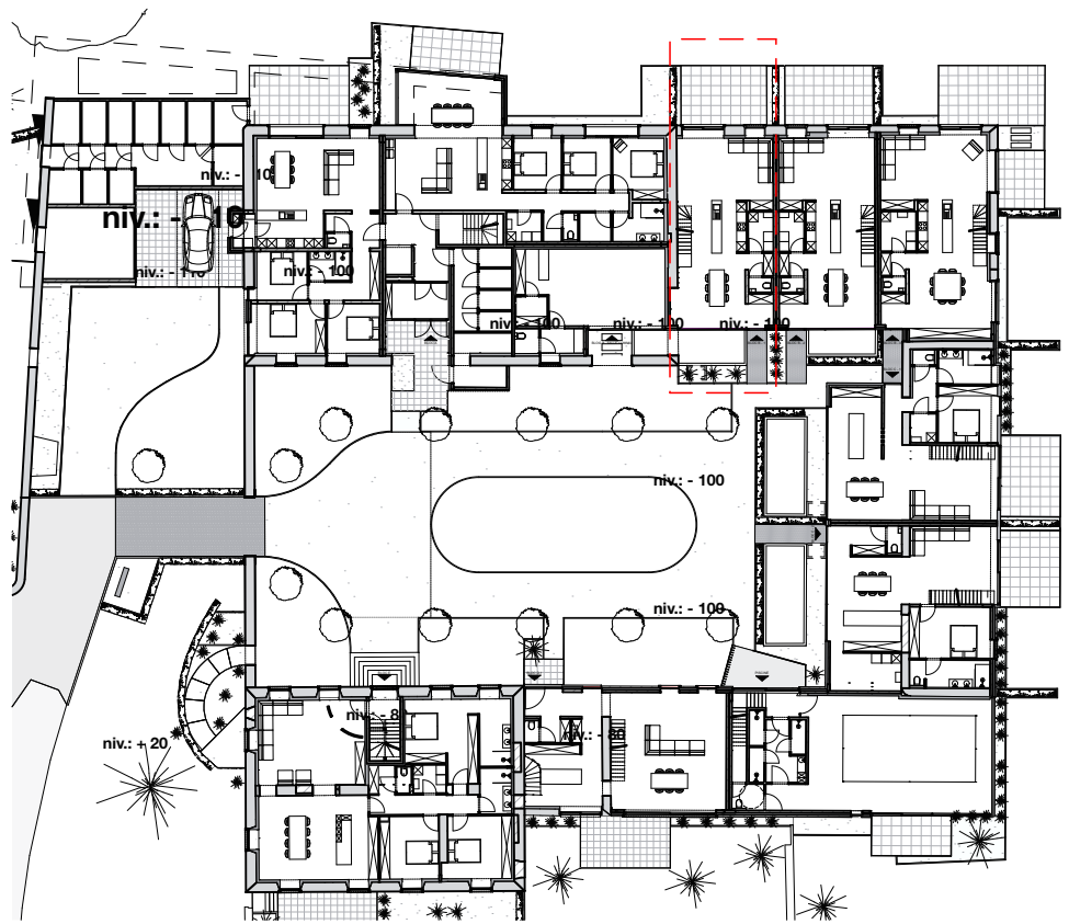
Rez-de-chaussée 1:500
