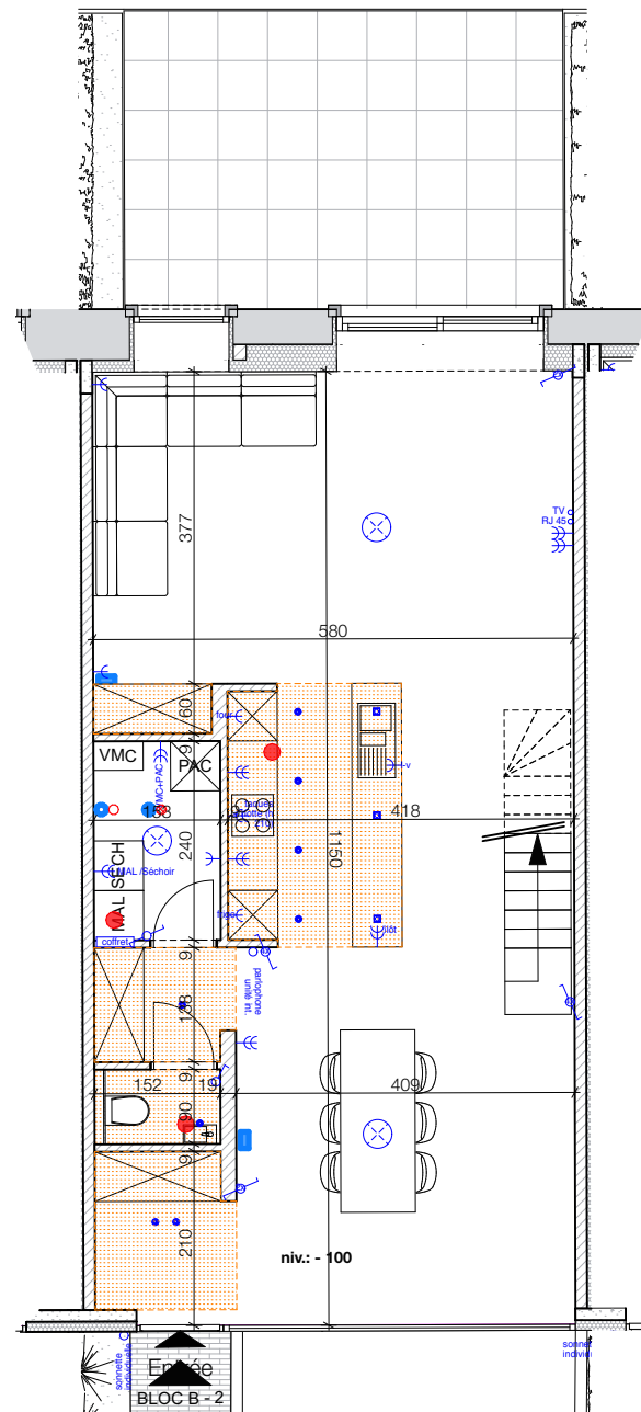
Rez-de-chaussée 1:100
