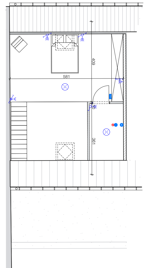
2ème étage 1:100
