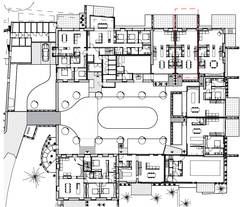
Rez-de-chaussée 1:500
