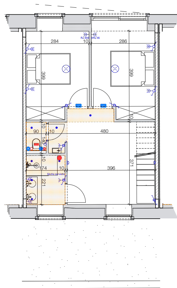
1er étage 1:100
