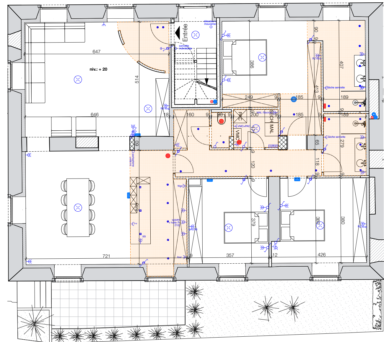
Rez-de-chaussée 1:100
