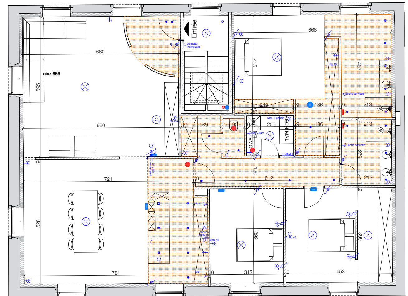
2ème étage
