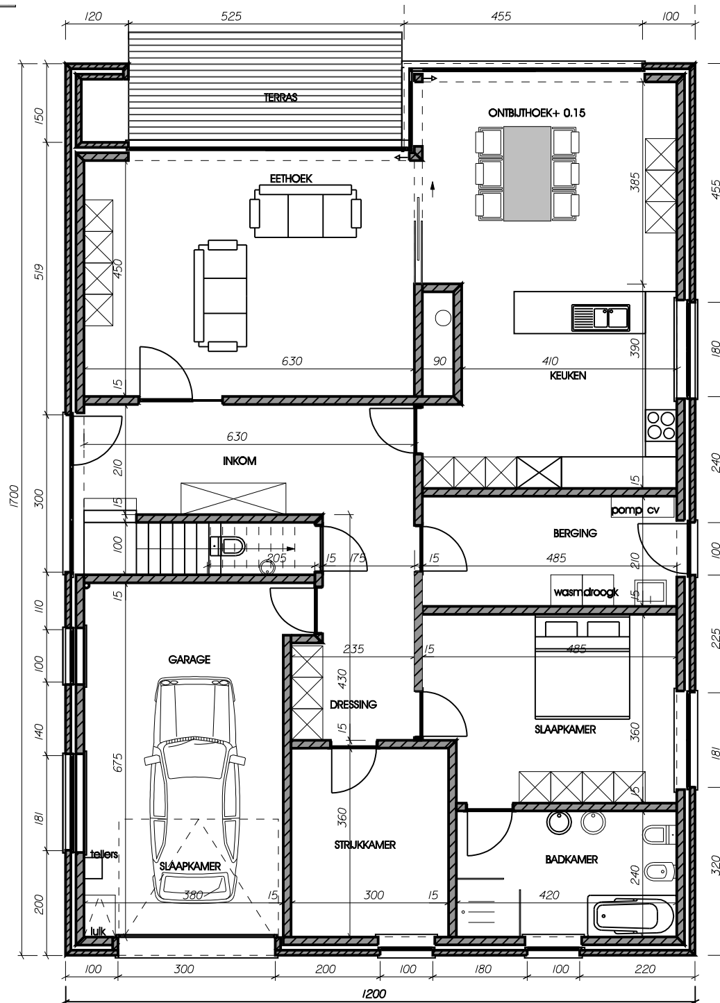
GRONDPLAN
