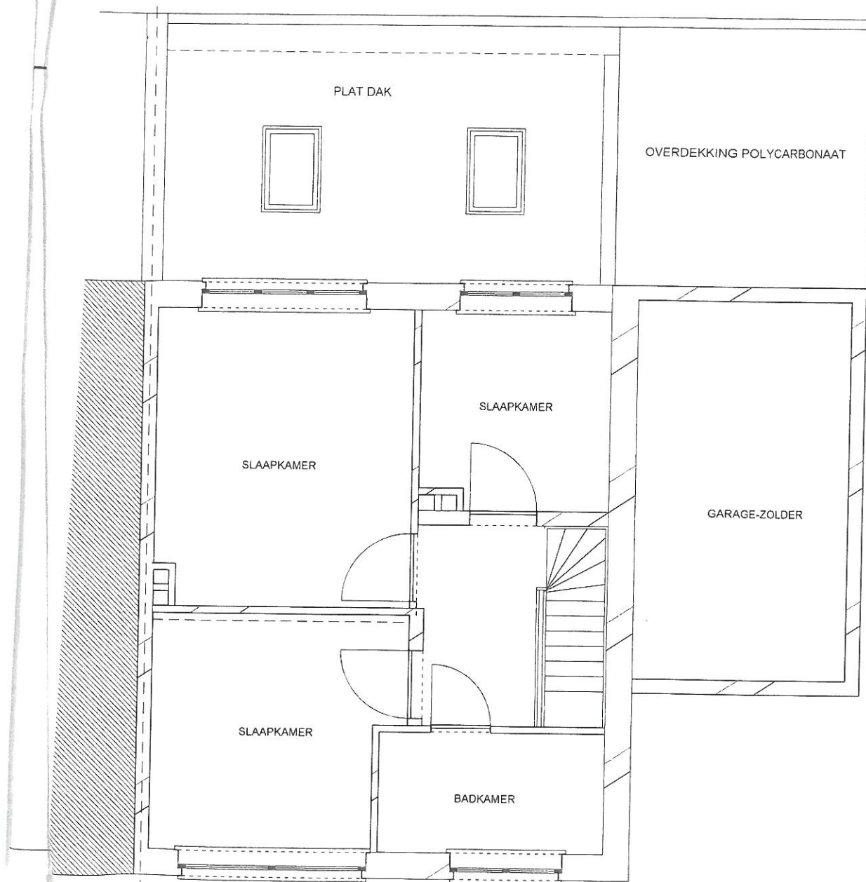
bestaande toestand VERDIEPING
