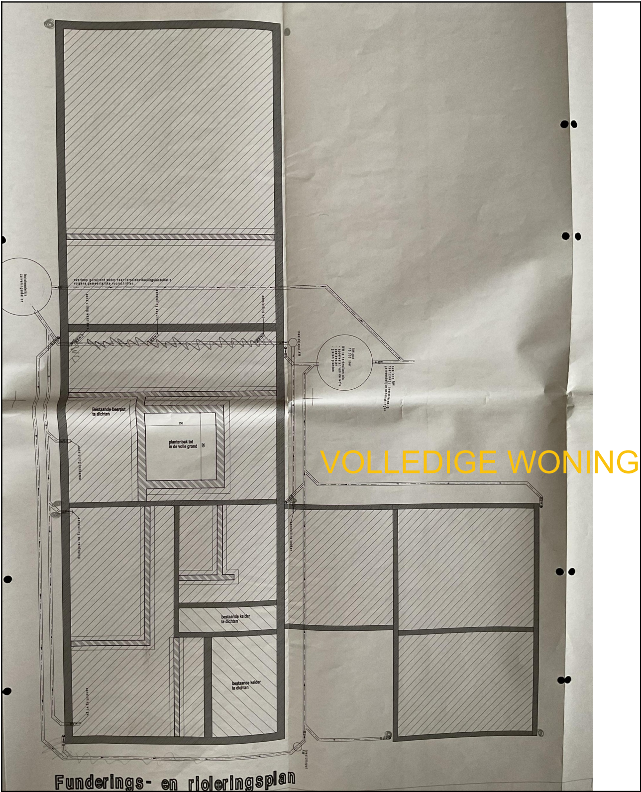
Legende van plan 1.4: Plan van de funderingen
