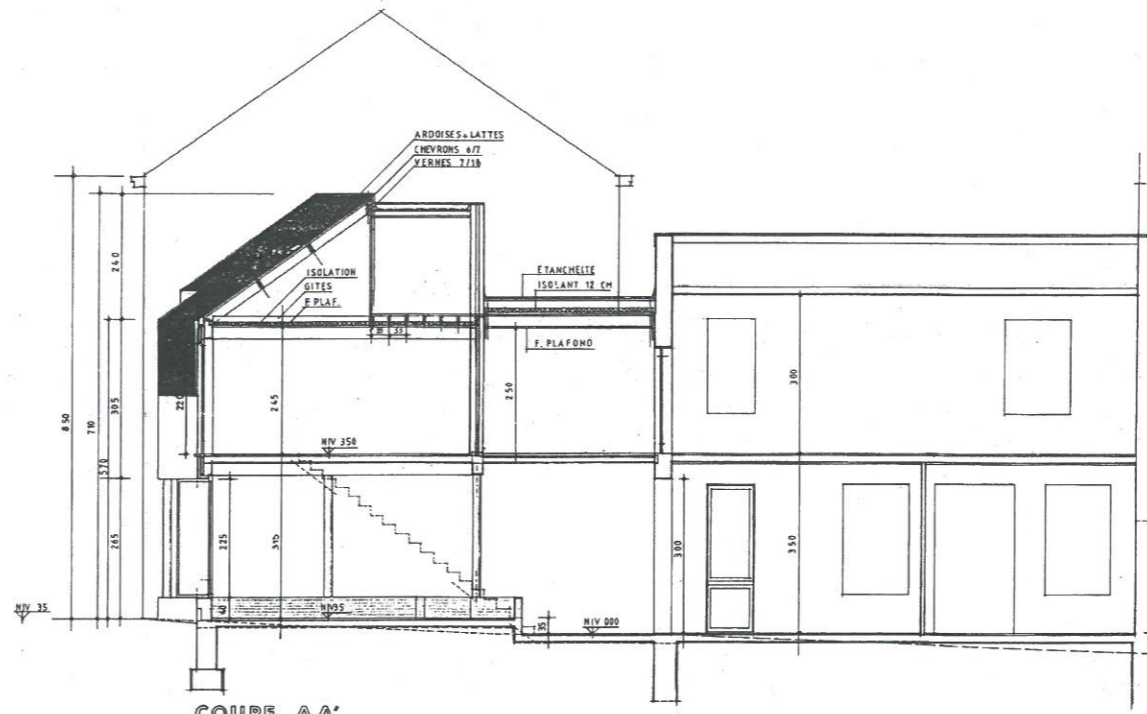
COUPE AA'
