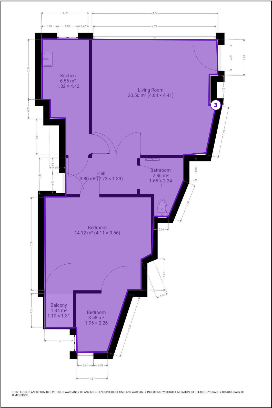
Legende van plan 1.3: GRONDPLAN NIV+2 VLOEREN
