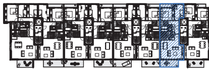
PLAN 3E ÉTAGE
