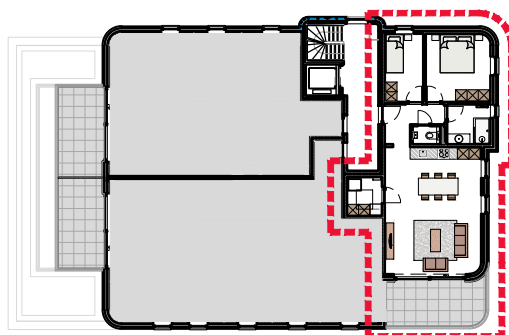
VERDIEPINGSPLAN
