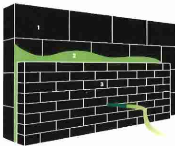
1. Dragende muur | 2. Ingeblazen isolatie | 3. Gevelsteen / gevelbekleding
