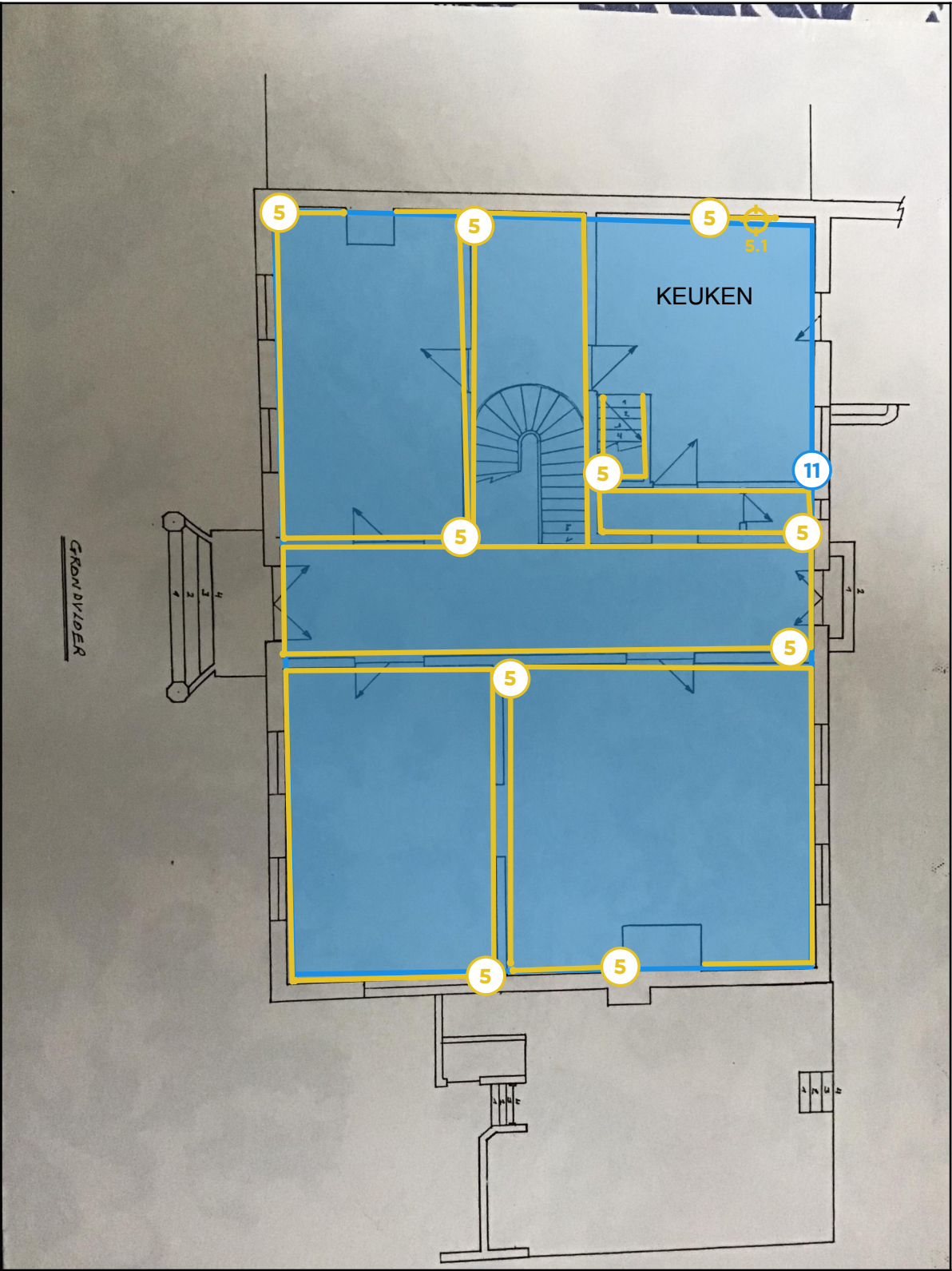
Legende van plan 1.3: Hoofdgebouw plan gelijkvloers pleisterwerk
