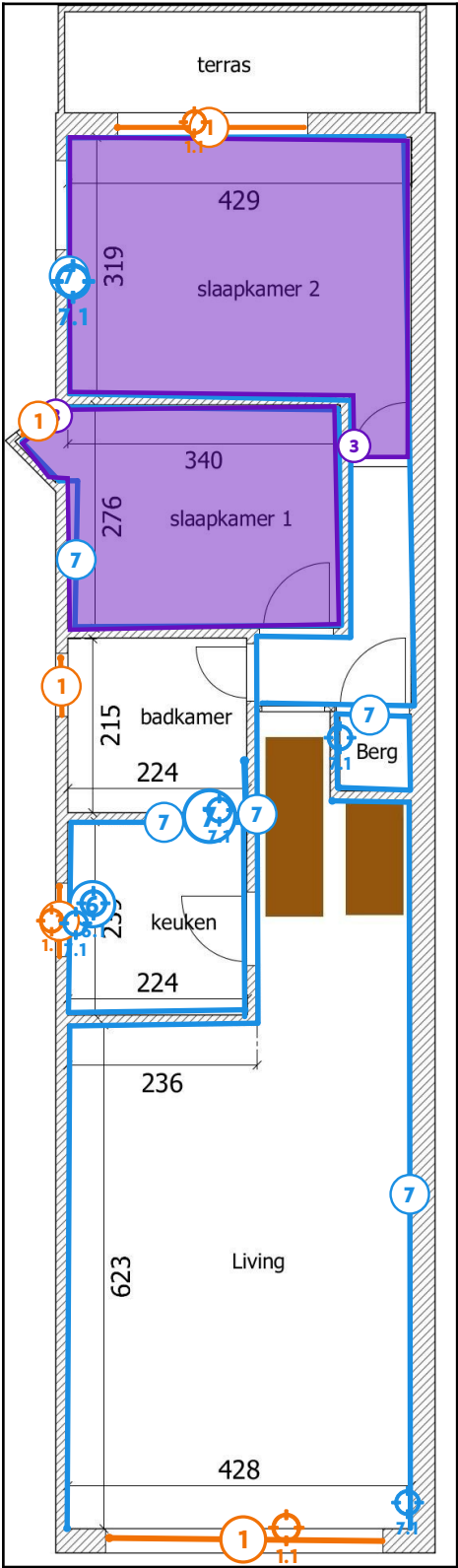
Legende van plan 1.3: plan appartement 0214
