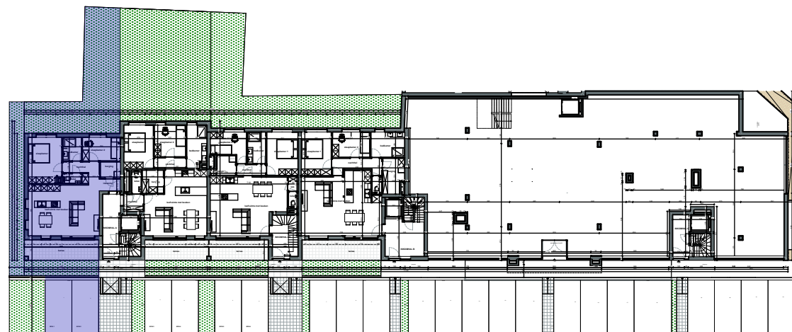
0 Gelijkvloers - B-A0.1 1:100
