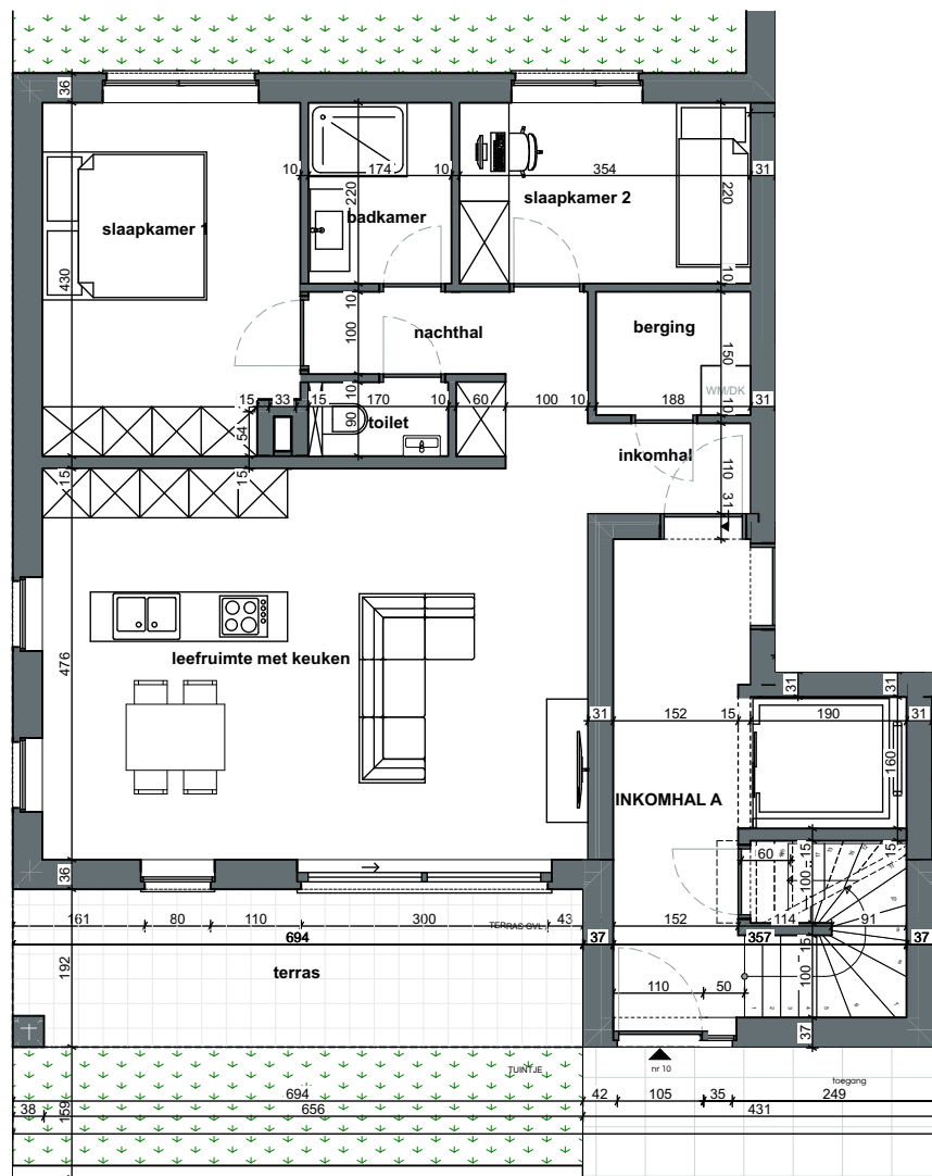
0 Gelijkvloers - B-A0.1 1:100
