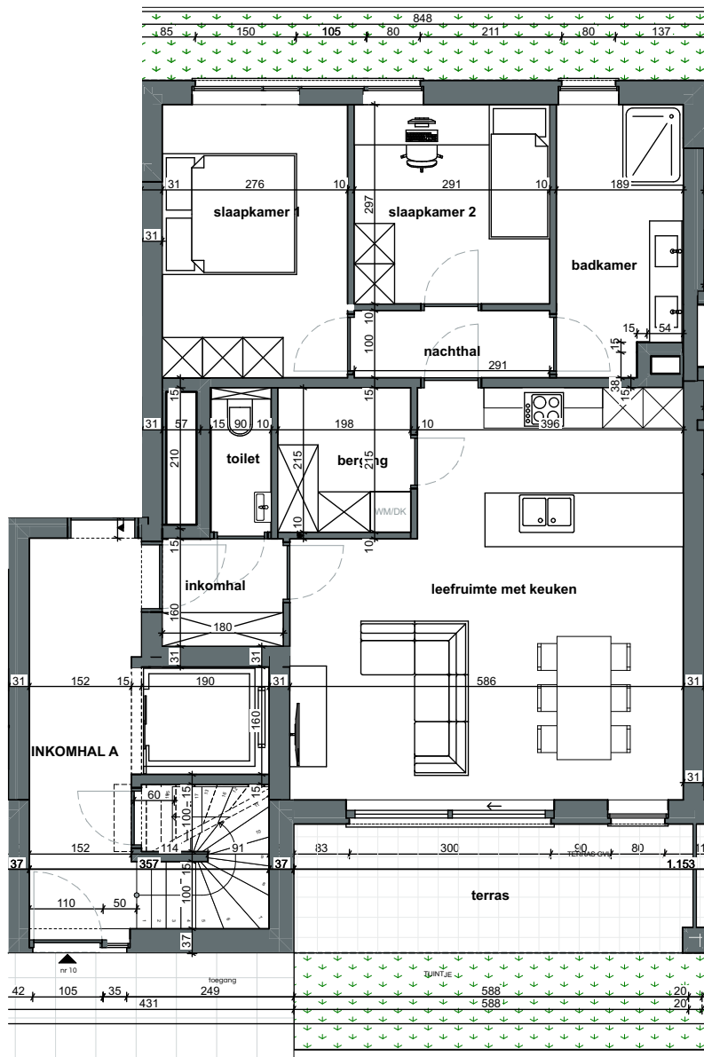
0 Gelijkvloers - B-A0.2 1:100
