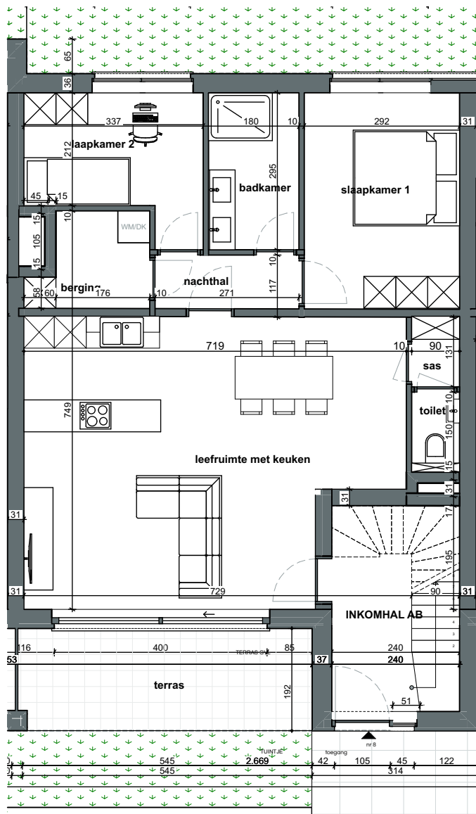
0 Gelijkvloers - B-AB0.1 1:100
