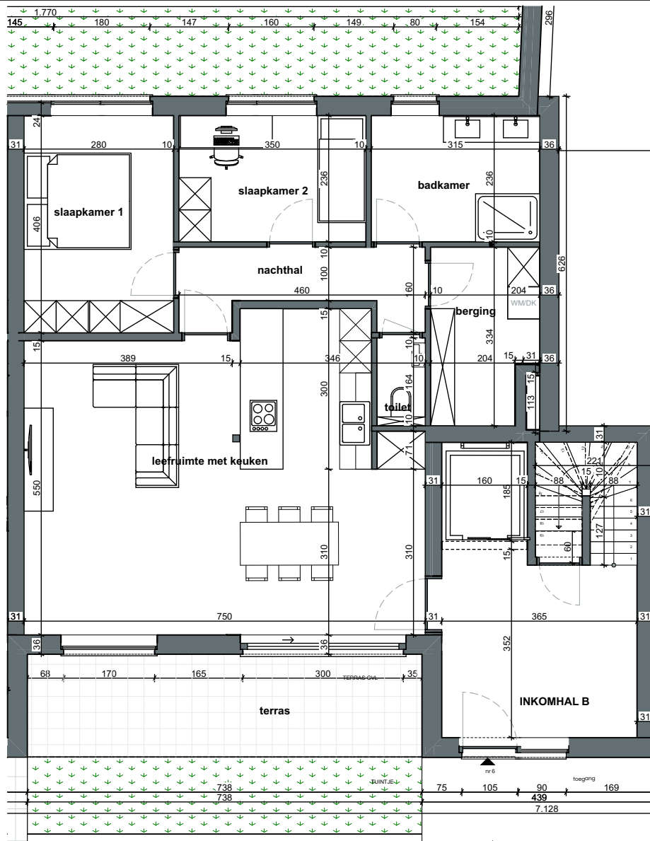
0 Gelijkvloers - B-B0.1 1:100
