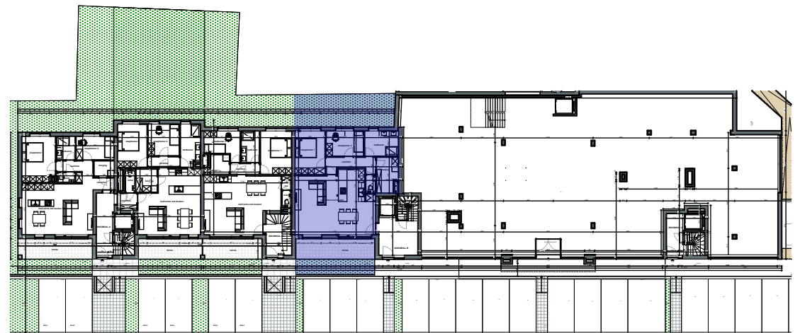
0 Gelijkvloers - B-B0.1 1:100
