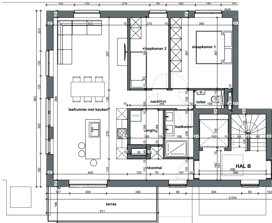
Verdieping 3 - B-B3.1
