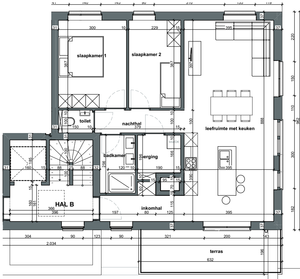
Verdieping 3 - B-B3.2 1:100
