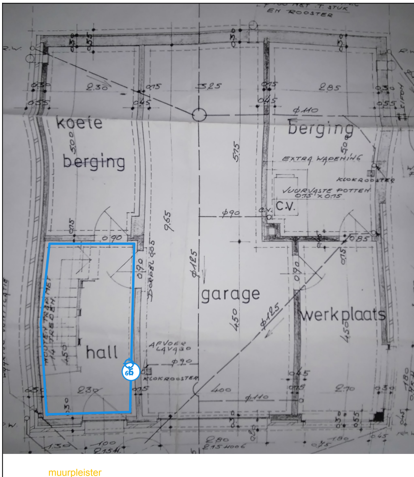
Legende van plan 1.1: Plan woning V-1
