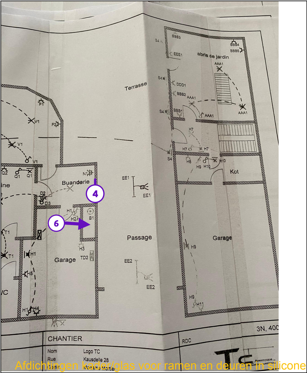
Legende van plan 1.2: GELIJKVLOERS - DEEL 2
