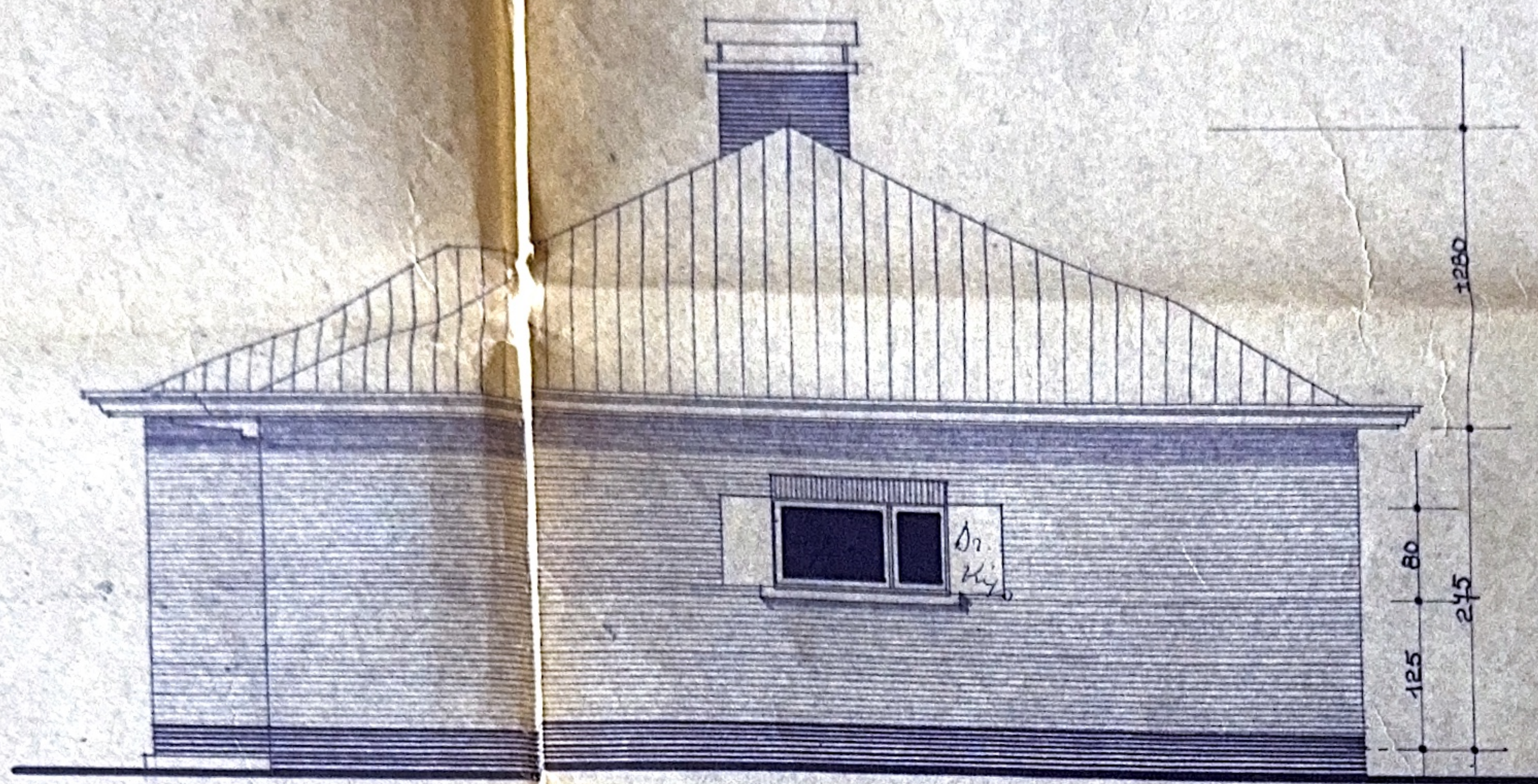
ZIJGEVEL RECHTS.
