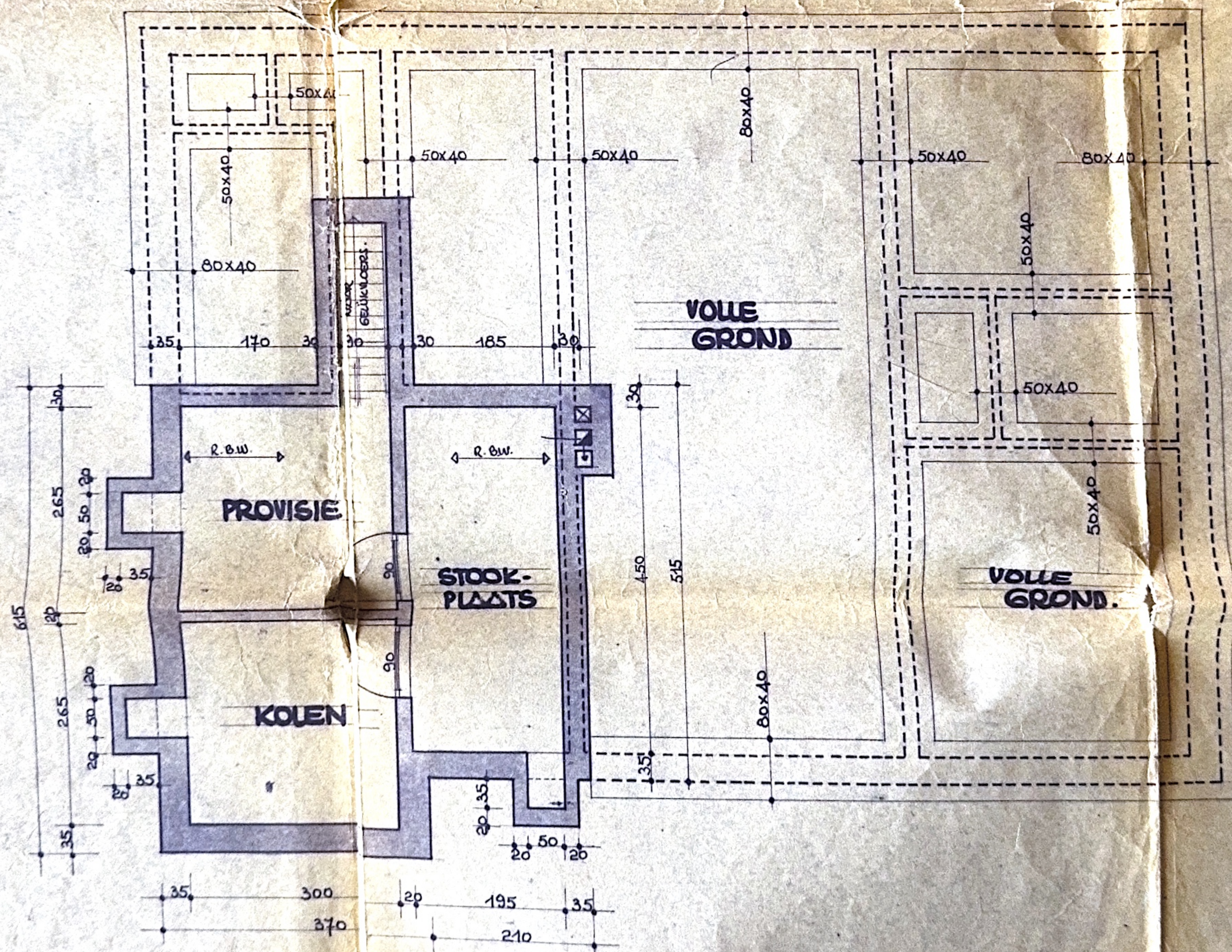
KELDERS & FUNDERINGEN.
