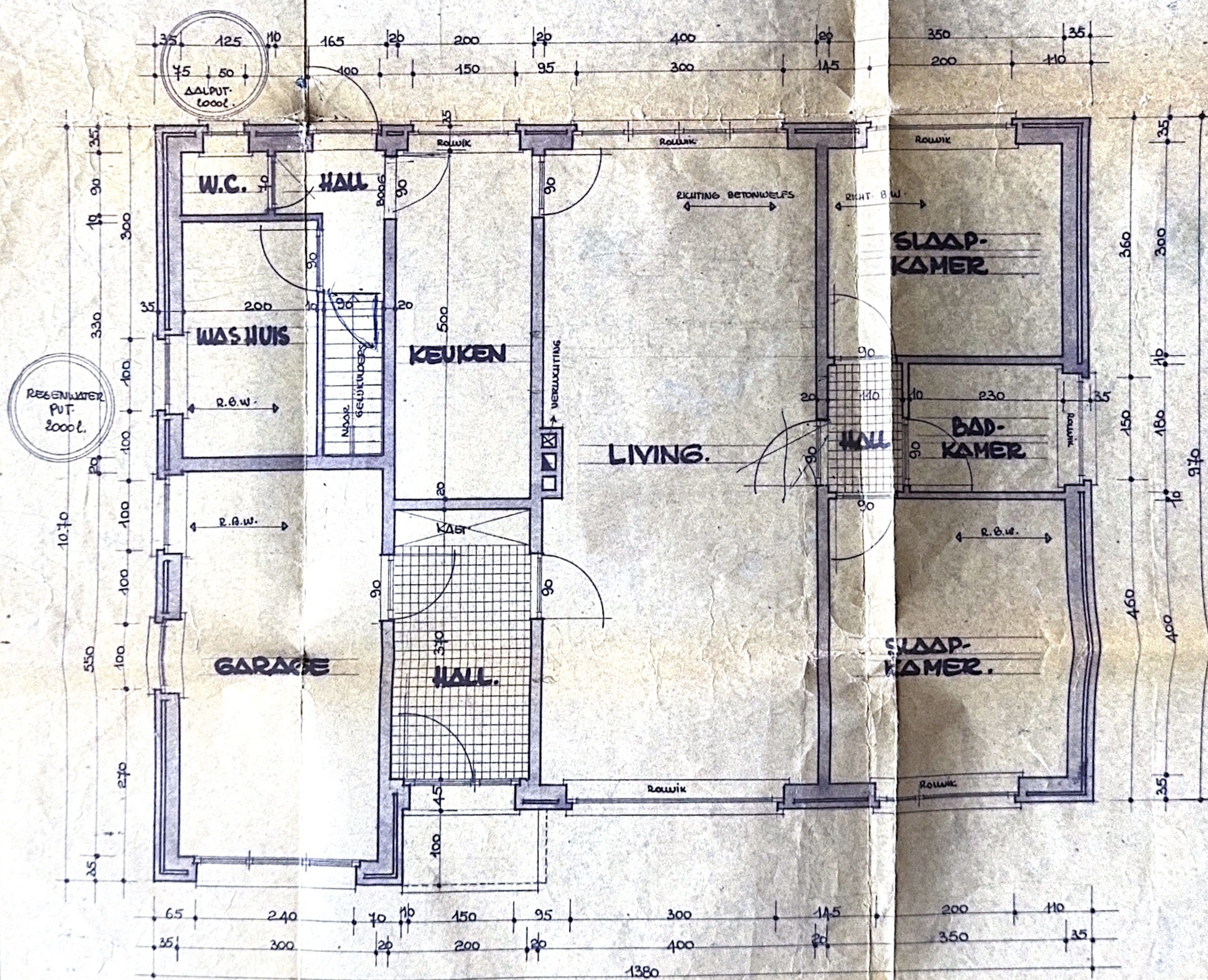
GELIJKVLOERS.
