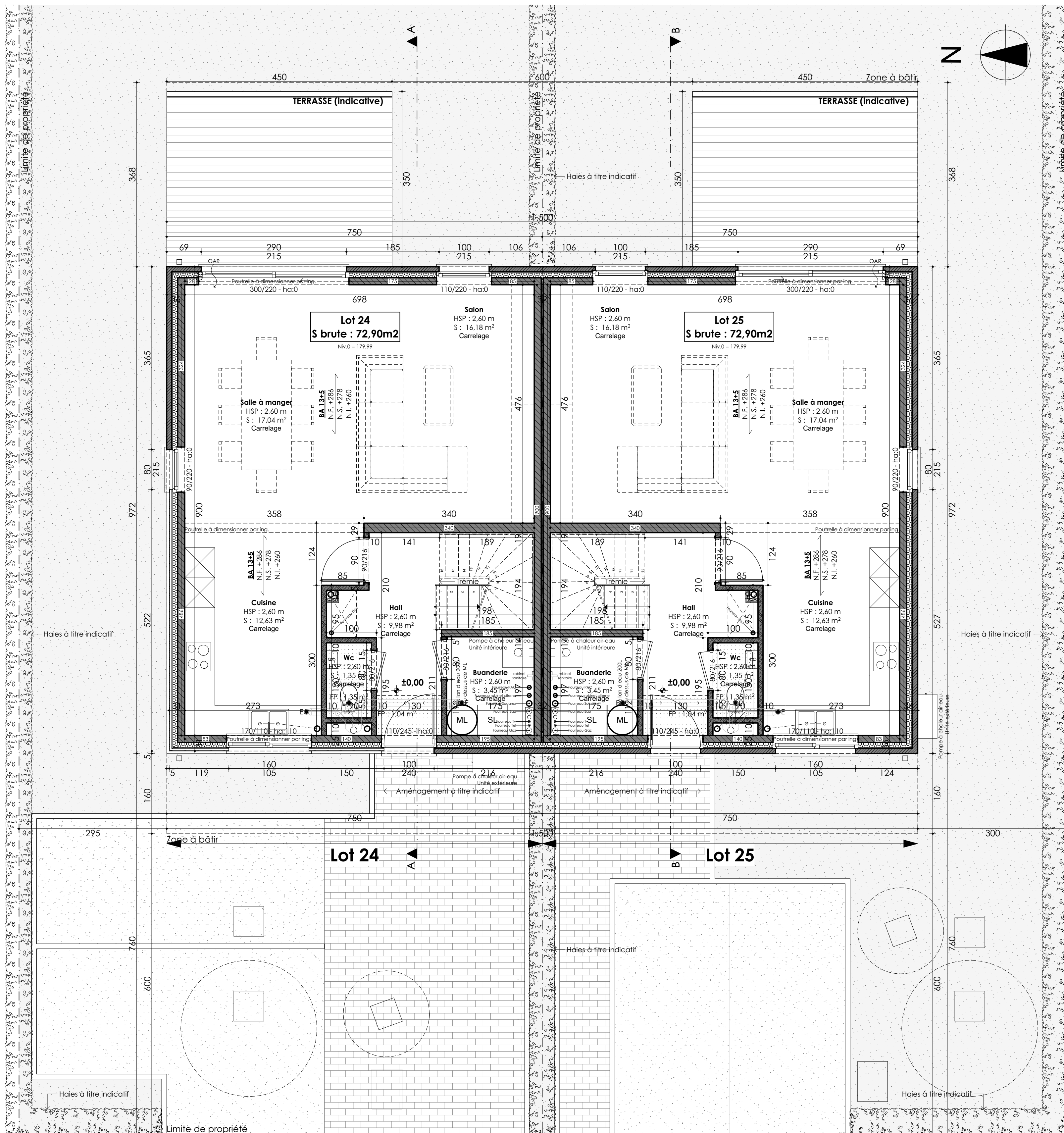
Plan du rez-de-chaussée
