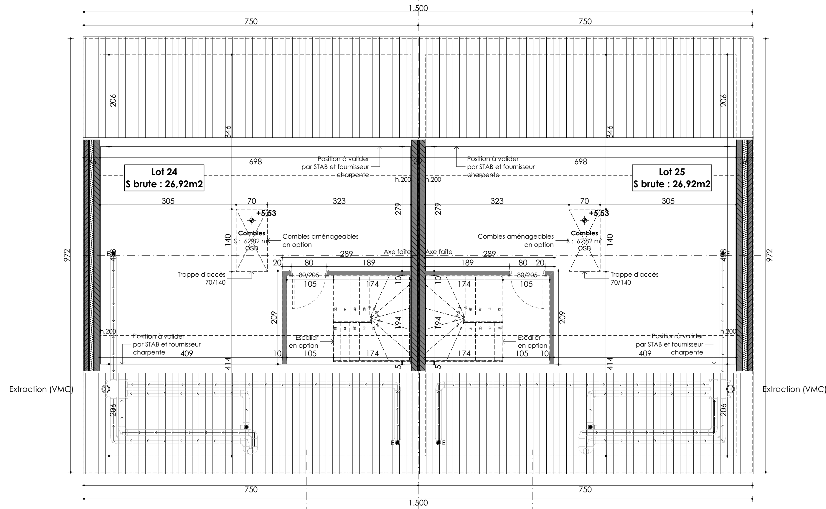
Plan des combles
