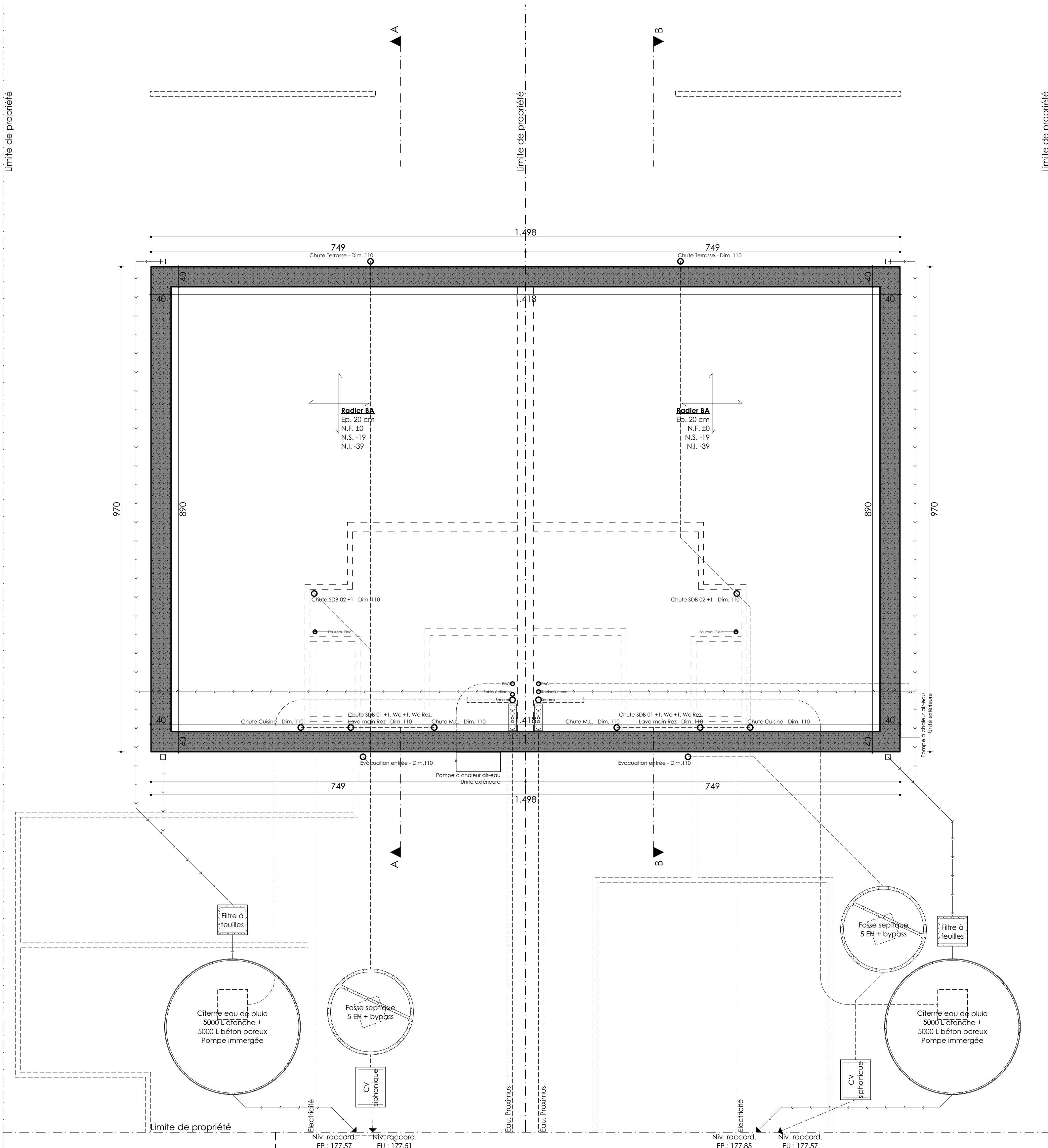
Plan du sous-sol
