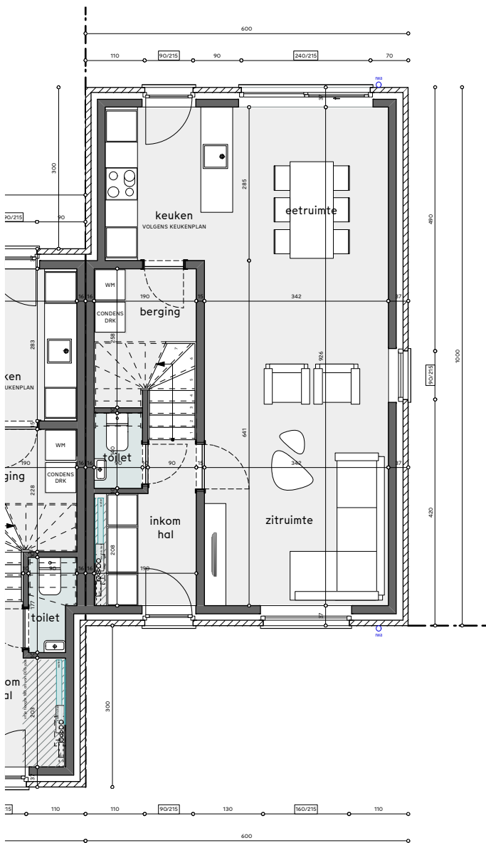
GRONDPLAN gelijkvloers
