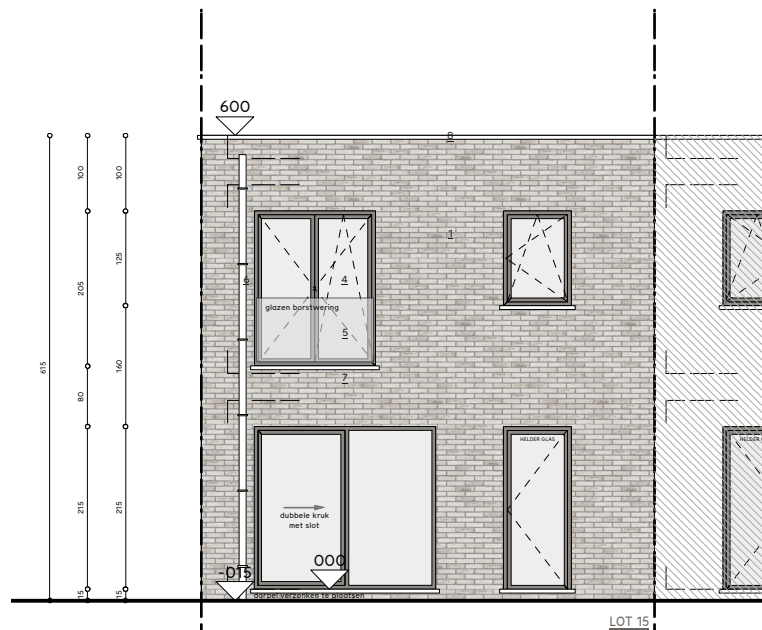
AANZICHT achtergevel
