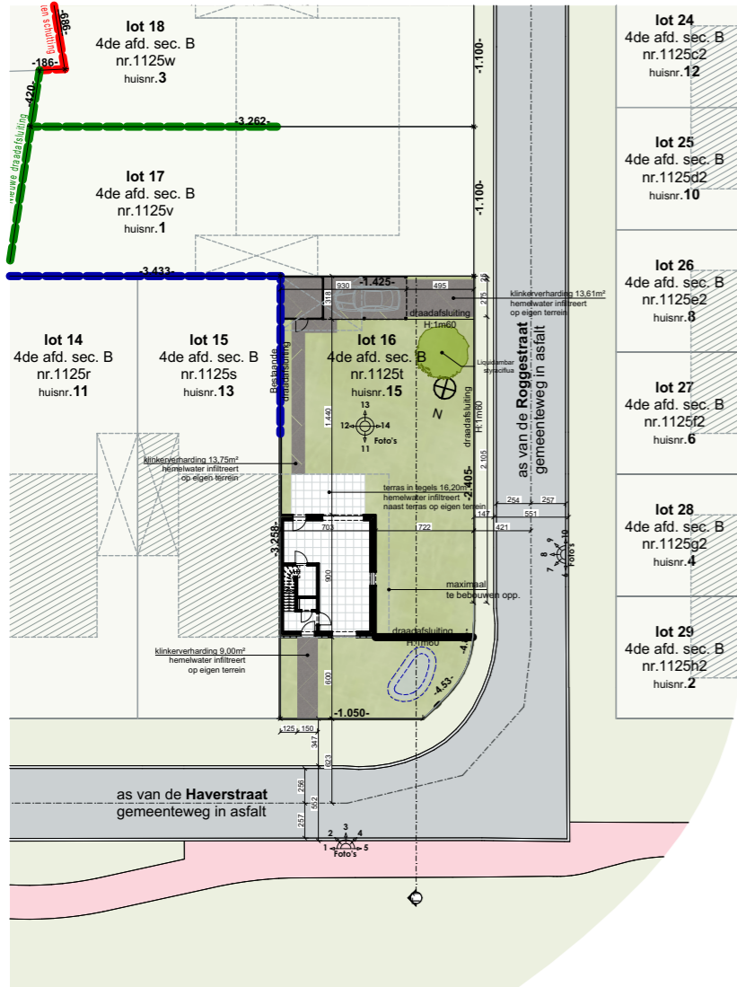
Gelijkvloers 1:100
