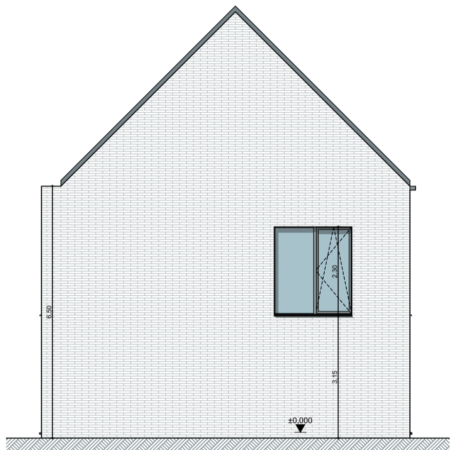
WONING 3: zijgevel links 1:100
