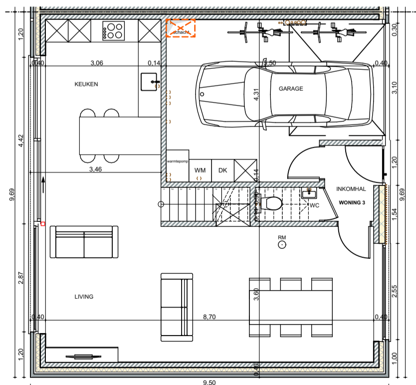
WONING 3: plan gelijkvloers 1:100
