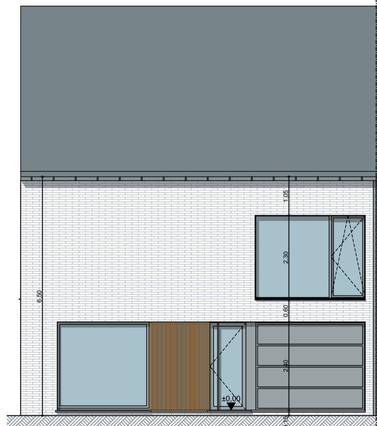
WONING 3: voorgevel 1:100
