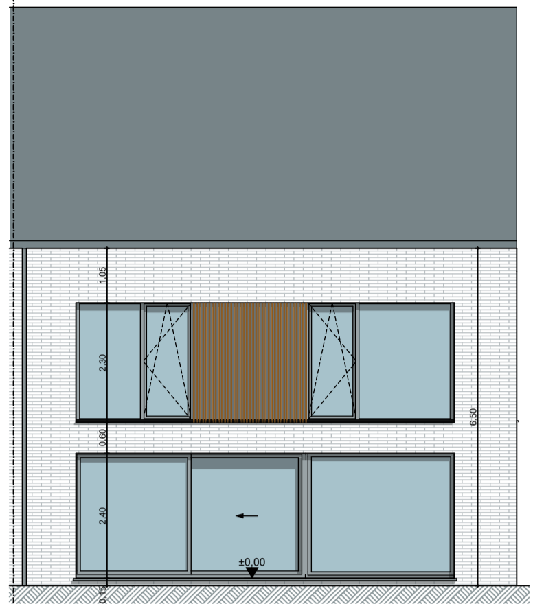
WONING 3: achtergevel 1:100
