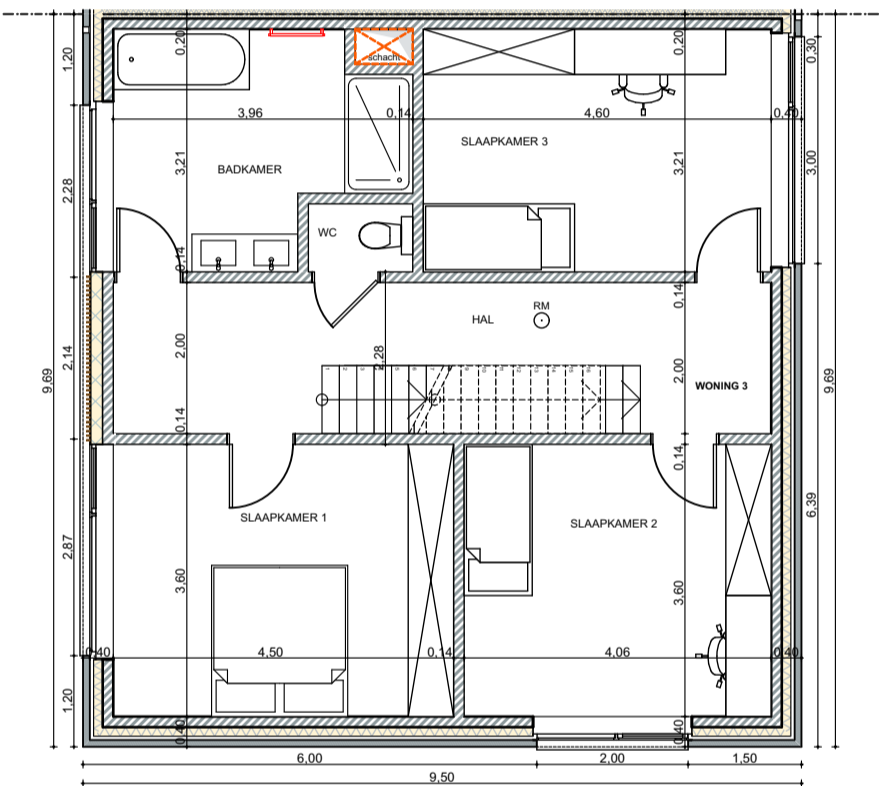
WONING 3: plan 1e verdieping 1:100
