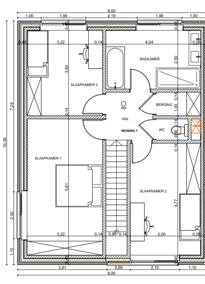
WONING 7: plan 1e verdieping 1:100
