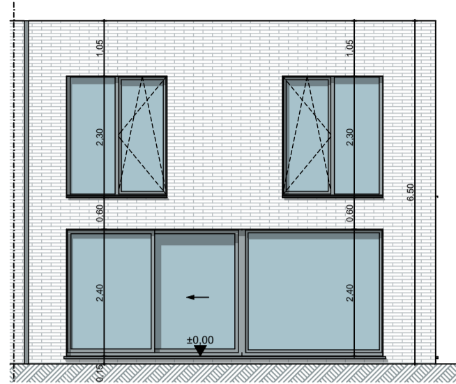
WONING 7: achtergevel 1:100
