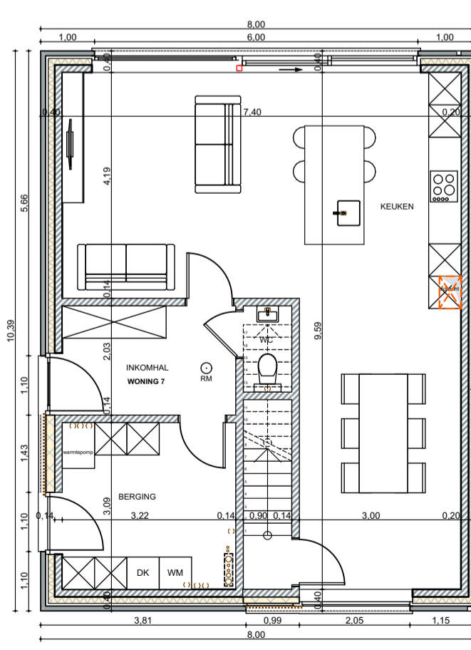
WONING 7: plan gelijkvloers 1:100
