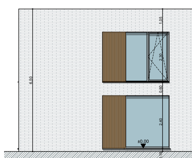
WONING 7: voorgevel 1:100
