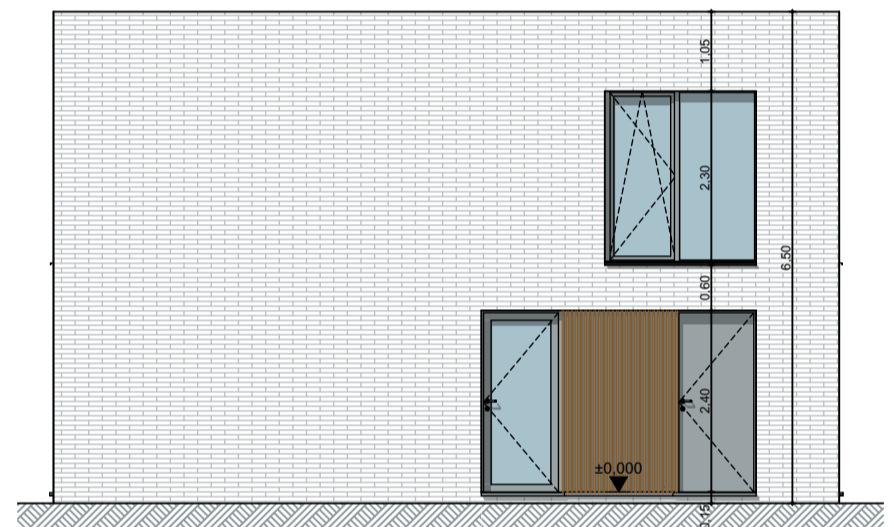
WONING 7: zijgevel links 1:100
