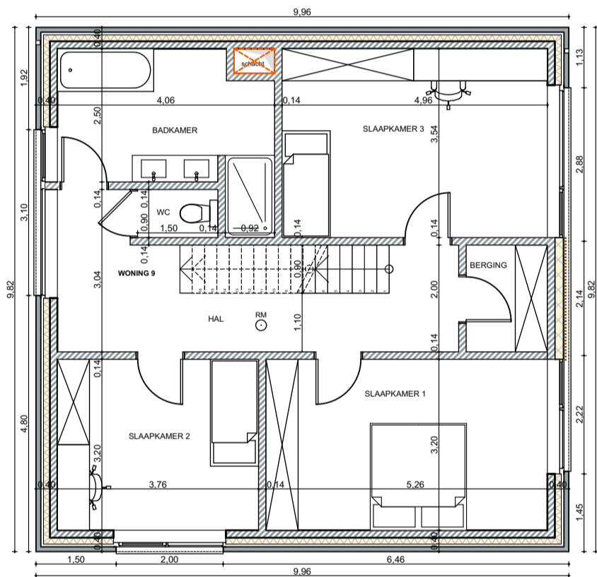
WONING 9: plan 1e verdieping 1:100
