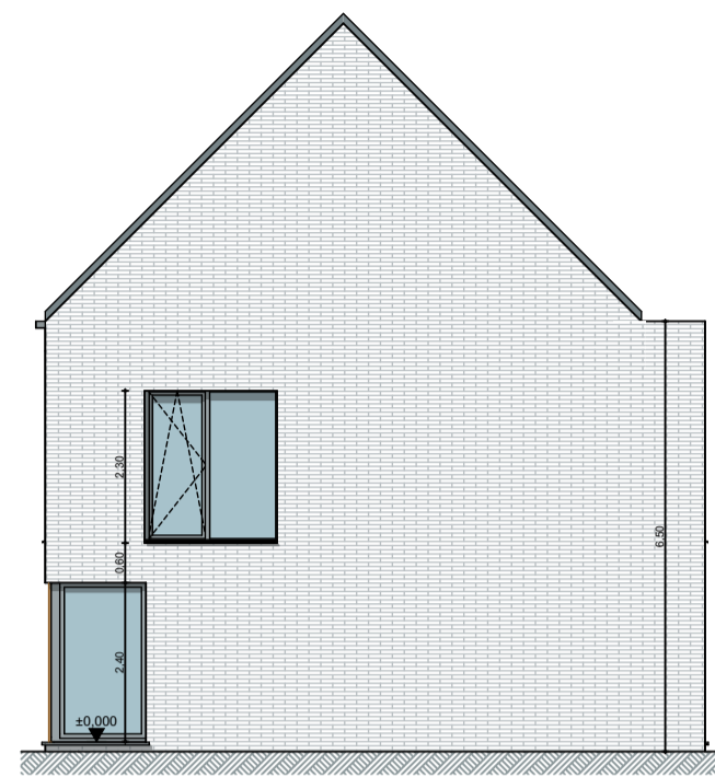
WONING 9: zijgevel rechts 1:125
