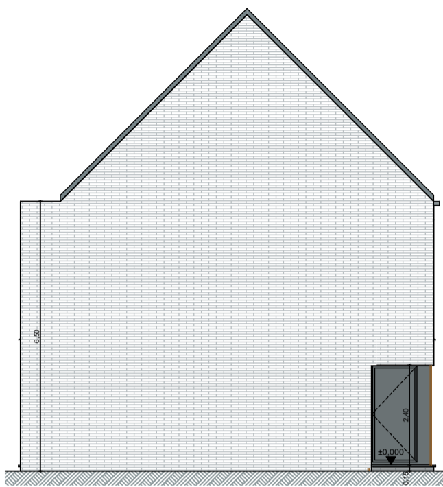
WONING 9: zijgevel links 1:125
