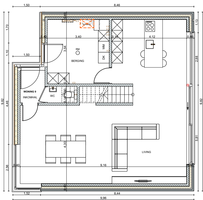
WONING 9: plan gelijkvloers 1:100
