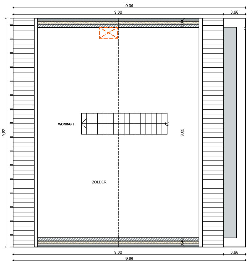
WONING 9: plan 2e verdieping 1:100
