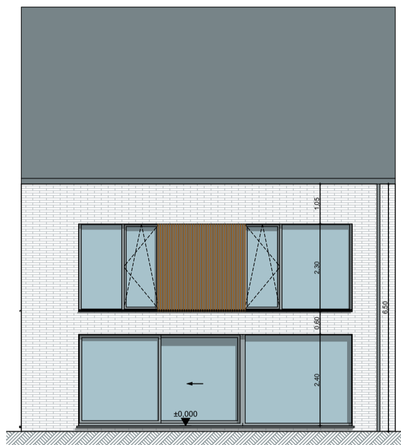
WONING 9: achtergevel 1:100
