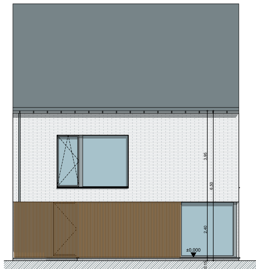
WONING 9: voorgevel 1:100
