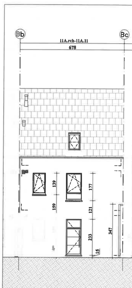
Façade Entrée
