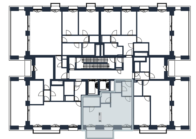
VERDIEPING +1
