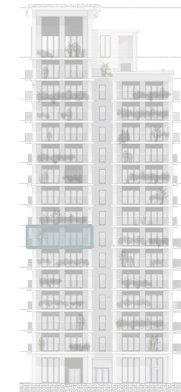
GEVEL NOORDWEST
