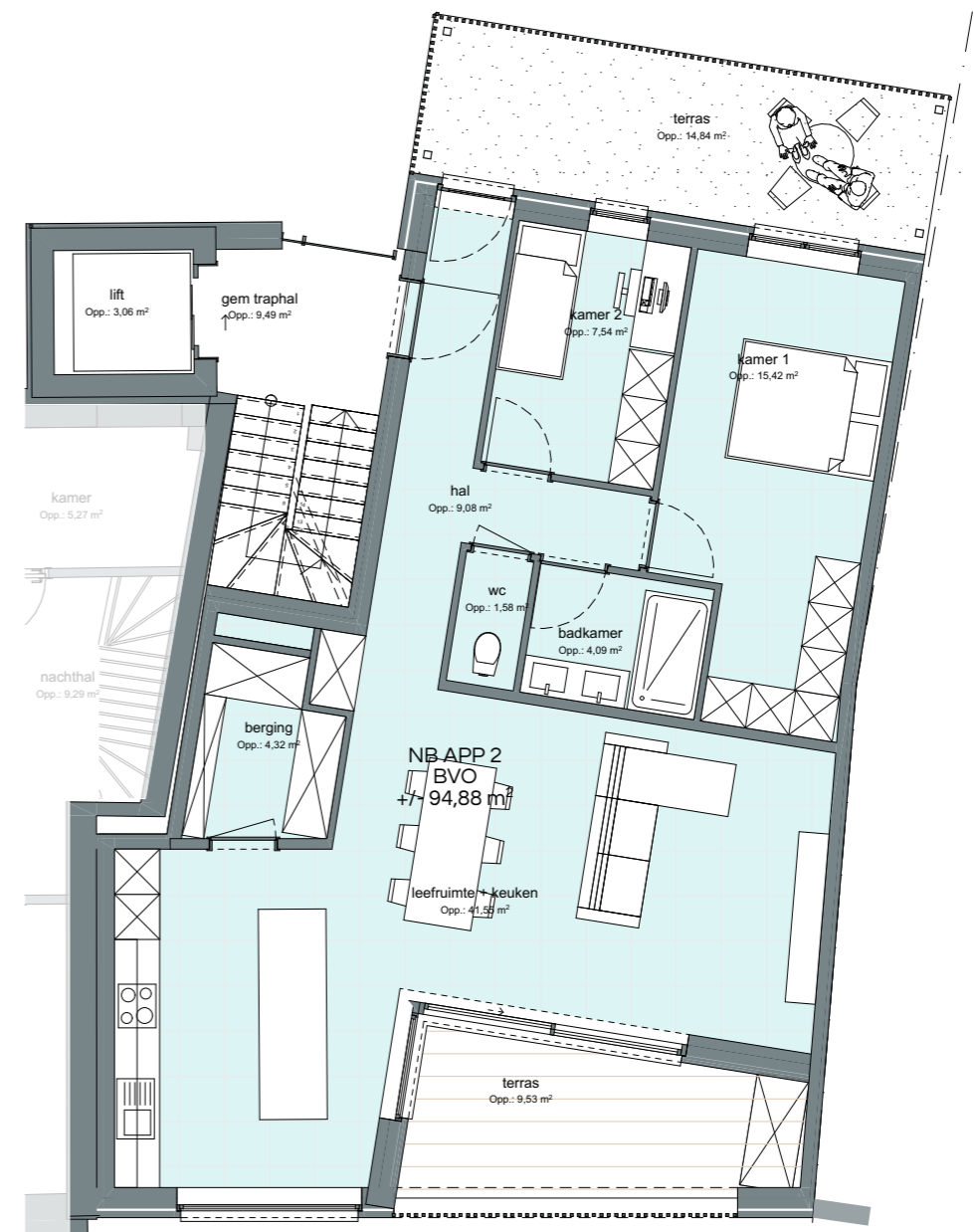
2e verdieping 1:100
