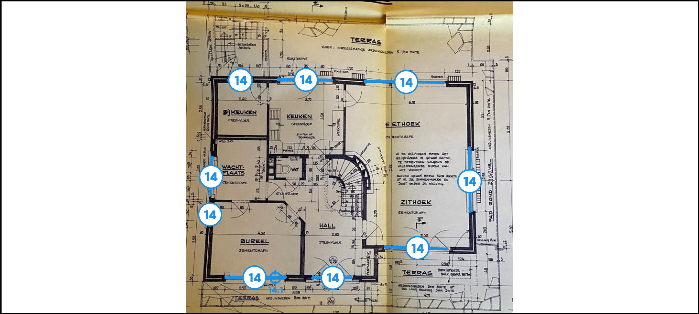
Legende van plan 1.5: Woning plan - Gelijkvloers
