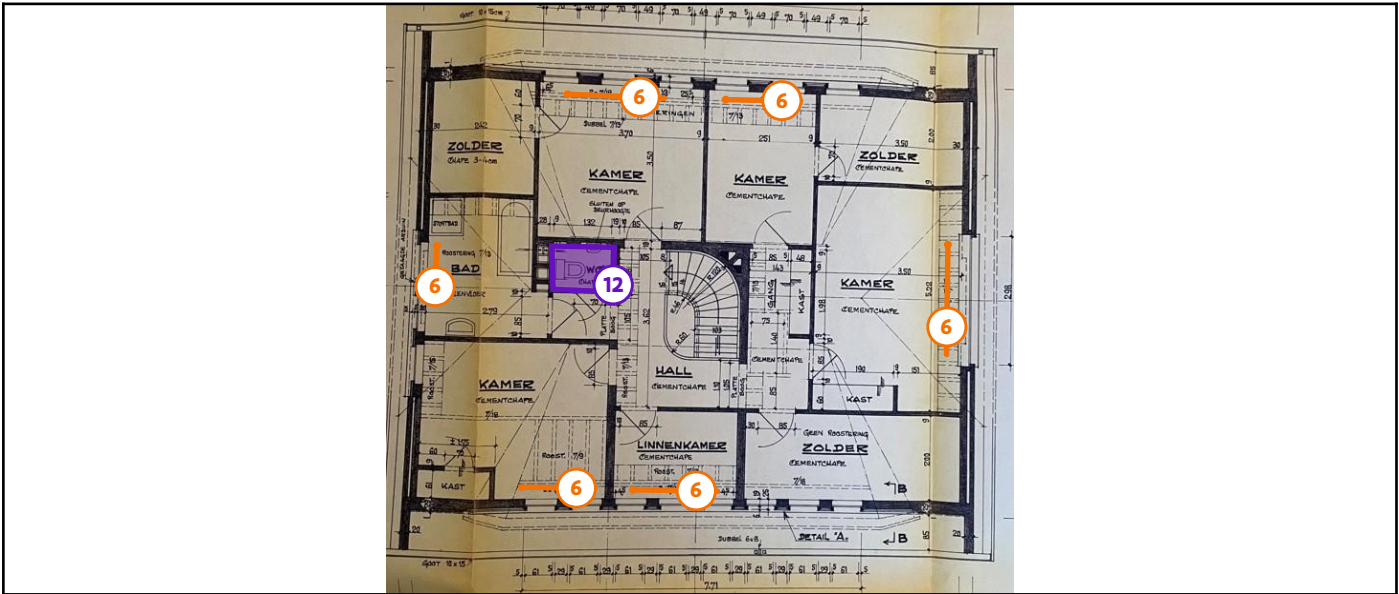
Legende van plan 1.8: Woning plan - Verdiep 1
