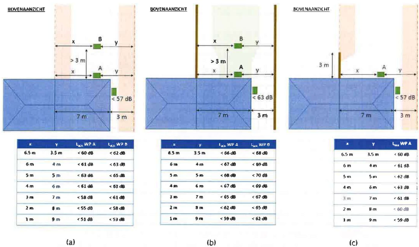
Figuur 13: Maximale geluidsvermogniveaus van de buitenunit voor diverse posities in de tuin (positie A en B) om te voldoen aan de vooropgestelde geluidsvoorwaarde van 45 dB(A) L_{Aeq,1min} overdag ter hoogte van de perceelsgrens. x is de afstand tot de linker perceelsgrens, y is de afstand tot de rechter perceelsgrens. De geluidsbron wordt verondersteld op 0,75 m (2/3 van de hoogte van de unit) en de geluidsdruk werd geëvalueerd op de perceelsgrens op 1,5 m hoogte. In situatie (a) zijn geen afsluitingen tussen de tuinen die een voldoende massa hebben om te zorgen voor afscherming. In situatie (b) is een volledig gesloten afsluiting met hoogte 1,8 m 27 en oppervlaktemassa \geq 10\text{kg/m}^2 rondom de volledige tuin, in situatie (c) is een volledig gesloten afsluiting met lengte 3 m, hoogte 1,8 m en oppervlaktemassa \geq 10\text{kg/m}^2 tussen de twee halfopen bebouwingen. Daarnaast wordt voor de 3 situaties ook het maximale geluidsvermogniveau weergegeven voor een buitenunit geplaatst bij de zijgevel op 3 m van de perceelsgrens.
