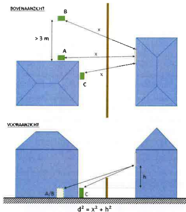
Figuur 11: Maximale geluidsvermogeniveaus van de buitenunit voor diverse posities in de tuin (positie A, B en C) om te voldoen aan de vooropgestelde geluidsvoorwaarde van 45 dB(A) L_{Aeq,1min} overdag ter hoogte van de opengaande ramen op de verdieping van de buurwoning. d is de afstand (in vogelvlucht) van de buitenunit tot het dichtstbijzijnde opengaande raam dat niet afgeschermd wordt door de afsluiting of het gebouw.
