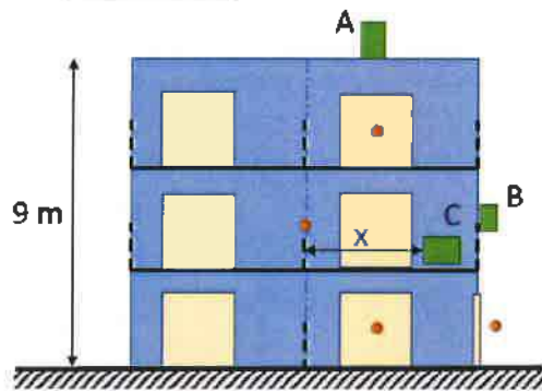
Figuur 19: Maximale geluidsvermogen-niveaus van de buitenunit van het appartement op de eerste verdieping voor een plaatsing op het dak (A), aan de gevel (B) of op het balkon (uit beton of massief hout) van het appartement (C) om te voldoen aan de vooropgestelde geluidsvoorwaarde 45 dB(A) L_{Aeq,1min} overdag. De geluidsdruk werd geëvalueerd voor de opengaande ramen en terrassen van de naburige appartementen. x is de afstand van de buitenunit tot het dichtstbijzijnde opengaande raam of een terras waar je kan verblijven.
