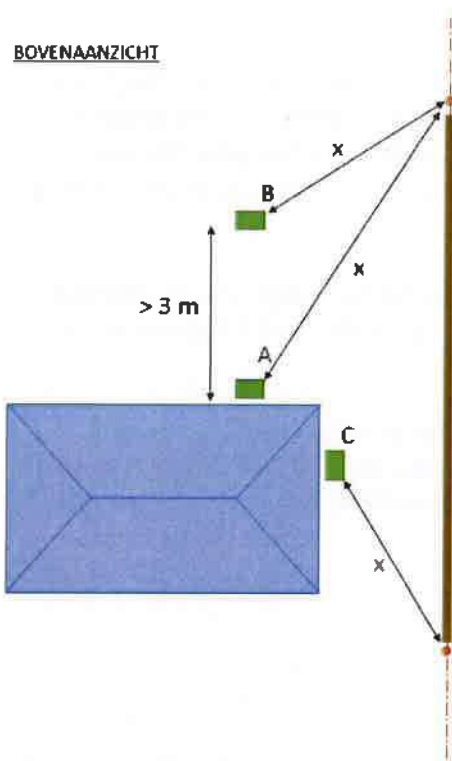
Figuur 12: Maximale geluidsvermogeniveaus van de buitenunit voor diverse posities in de tuin (positie A, B en C) om te voldoen aan de vooropgestelde geluidsvoorwaarde van 45 dB(A) L_{Aeq,1min} overdag op de perceelsgrens. x is de afstand van de buitenunit tot het dichtstbijzijnde punt op de perceelsgrens zonder afsluiting.
