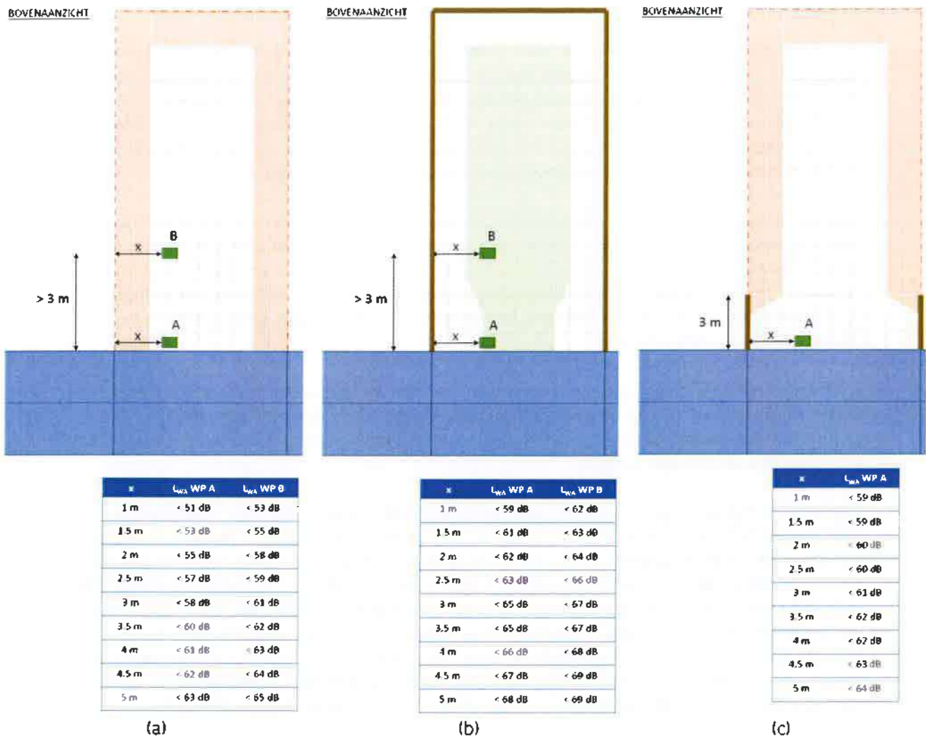
Figuur 15: Maximale geluidsvermogen-niveaus van de buitenunit voor diverse posities in de achtertuin (positie A en B 35 ) om te voldoen aan de vooropgestelde geluidsvoorwaarde 45 dB(A) L_{Aeq,1min} overdag. x is de kleinste afstand tot de dichtstbijzijnde perceelsgrens. De geluidsbron wordt verondersteld op 0,75 m (2/3 van de hoogte van de unit) en de geluidsdruk werd geëvalueerd op de perceelsgrens op 1,5 m hoogte. In situatie (a) zijn geen afsluitingen tussen de tuinen die een voldoende massa hebben om te zorgen voor afscherming. In situatie (b) is een volledig gesloten afsluiting met hoogte 1,8m en oppervlaktemassa \geq 10\text{kg/m}^2 rondom de volledige tuin 36 en in situatie (c) zijn volledig gesloten afsluitingen met lengte 3 m, hoogte 1,8 m en oppervlaktemassa \geq 10\text{kg/m}^2
