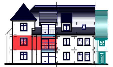
GEVEL / FAÇADE
