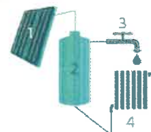
1 Zonnecollector | 2 Opslagvat zonneboiler | 3 Sanitair warm water | 4 Afhijf-element voor ruimteverwarming (radiateur)
