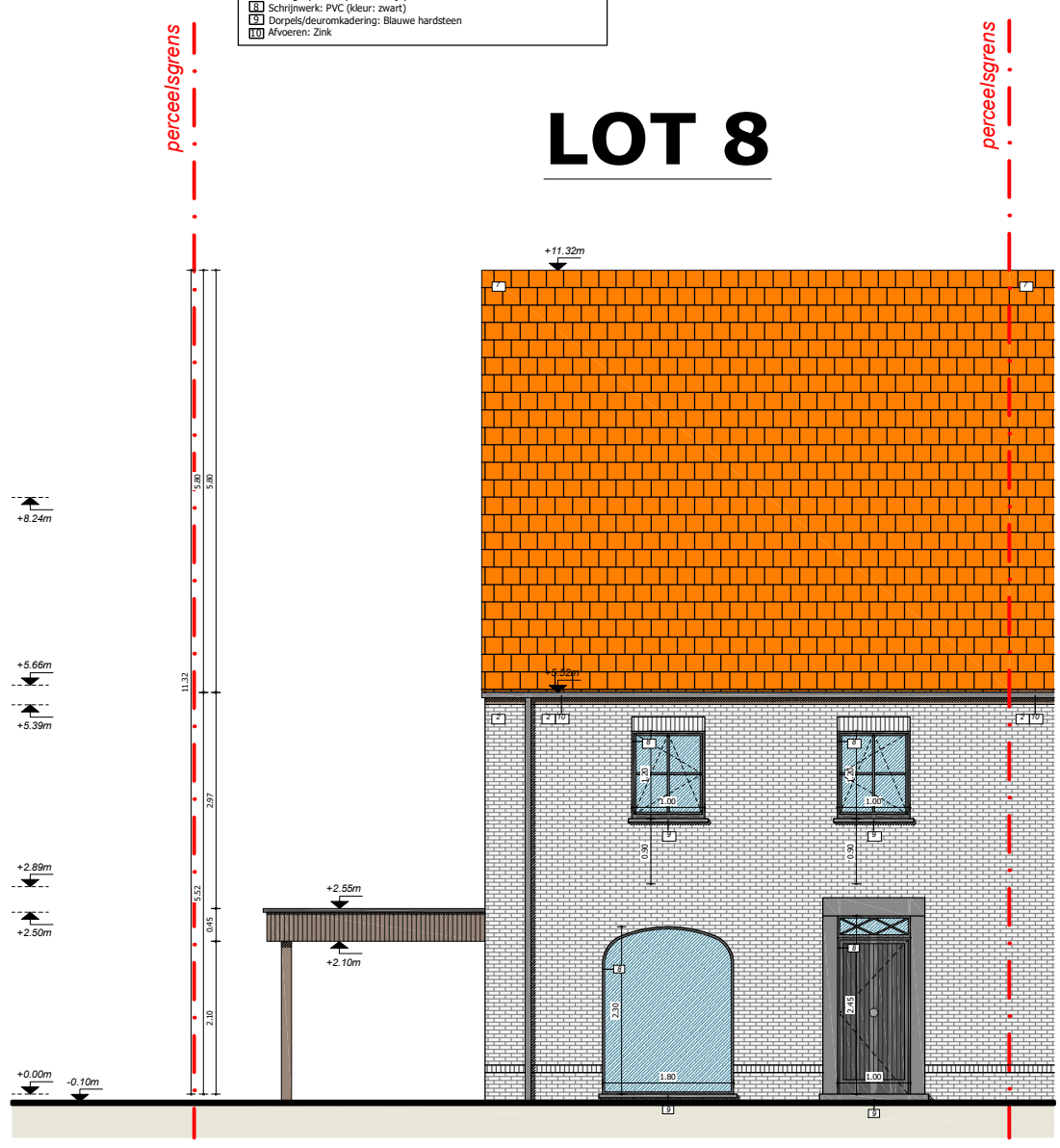
VOORGEVEL SCHAAL 1:100
