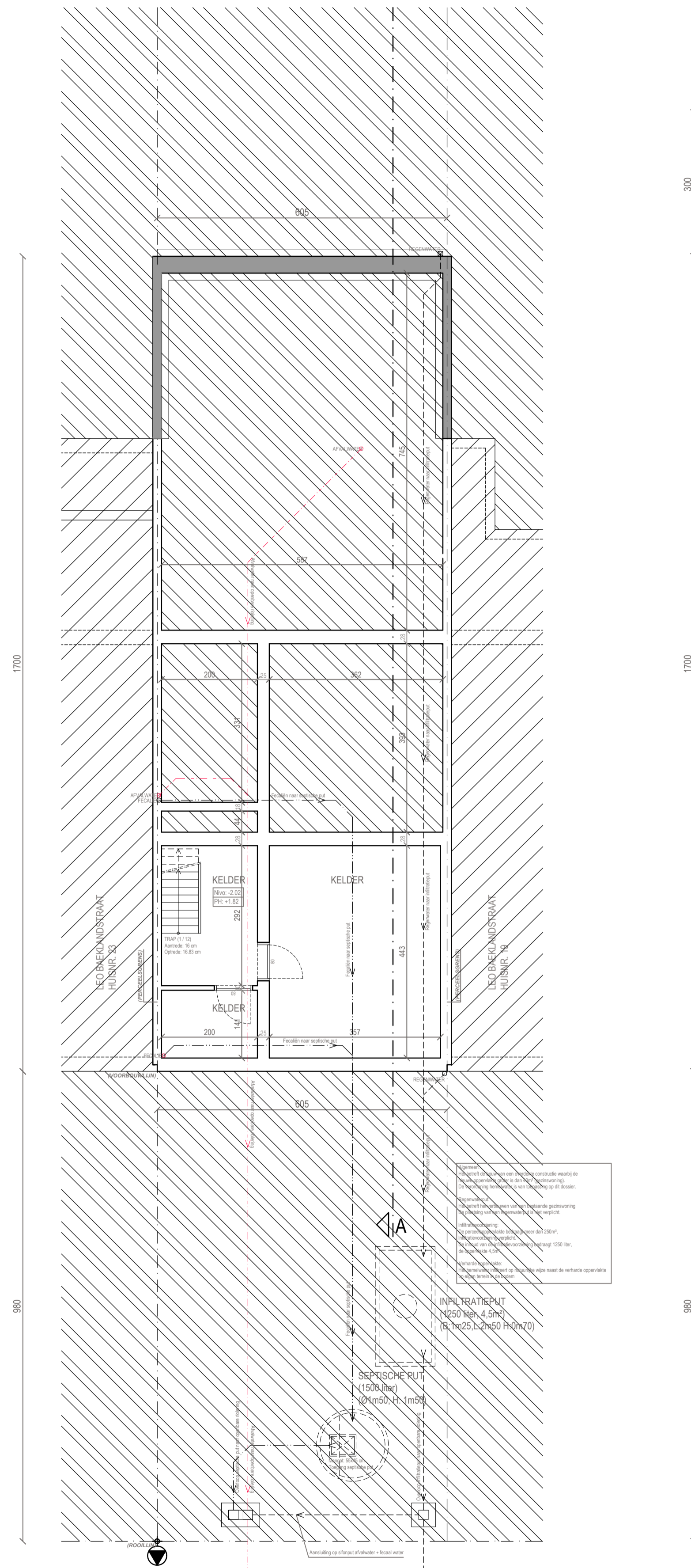
Nivo -1 (nieuwe toestand) (schaal 1/50)
