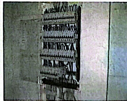
Coffret divisionnaire équipé et câblé
