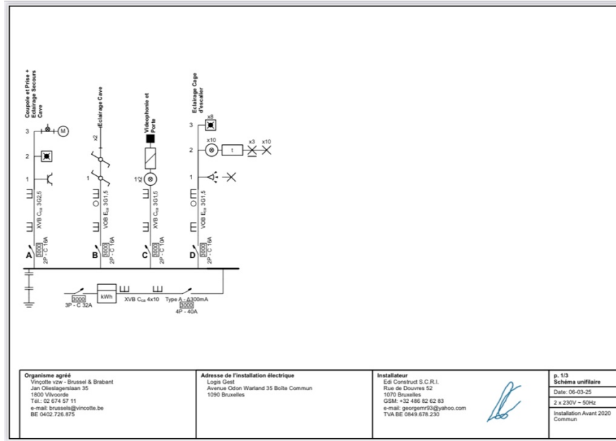
( Schémas unifilaires et plans de position )
