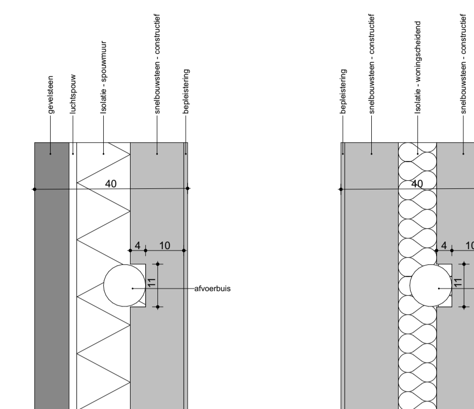
1:10 detail afvoer in muur
