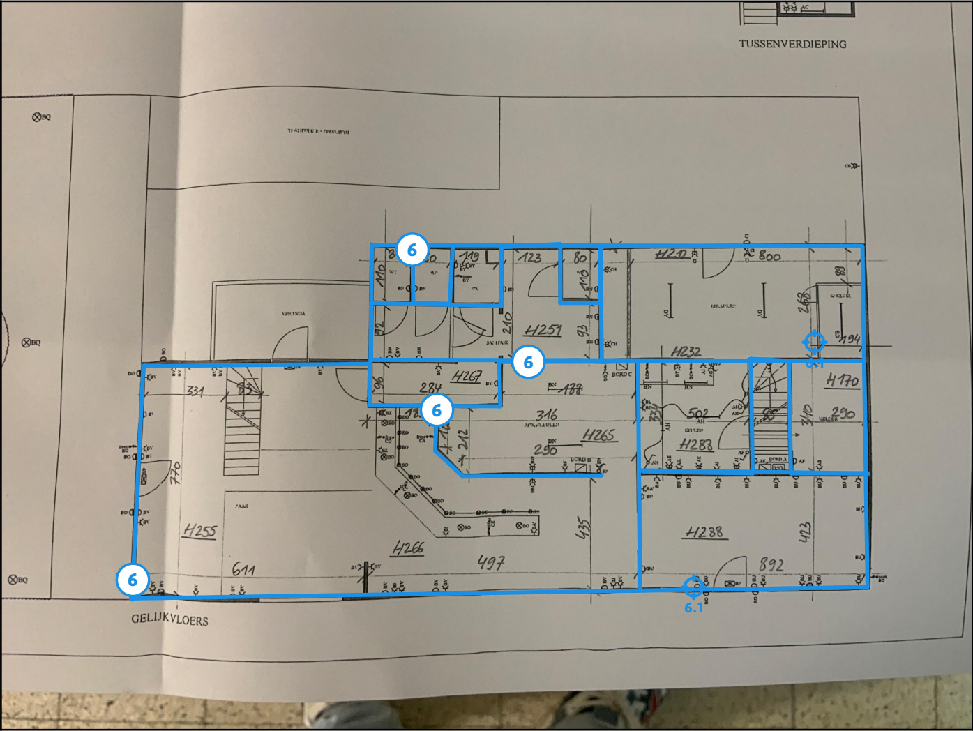
Legende van plan 1.2: gelijkvloers pleisterwerk muren plan
