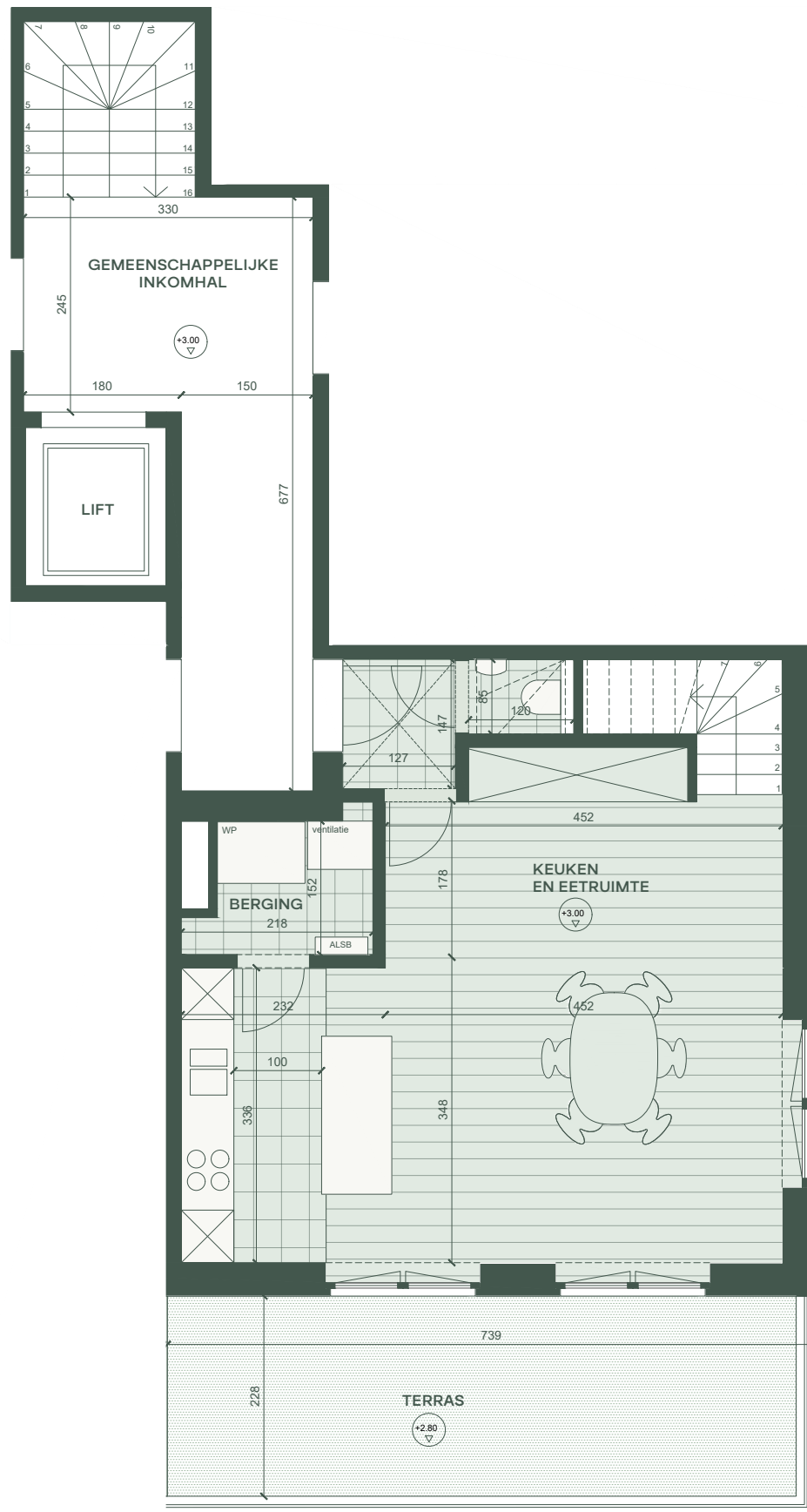
Niveau +1
